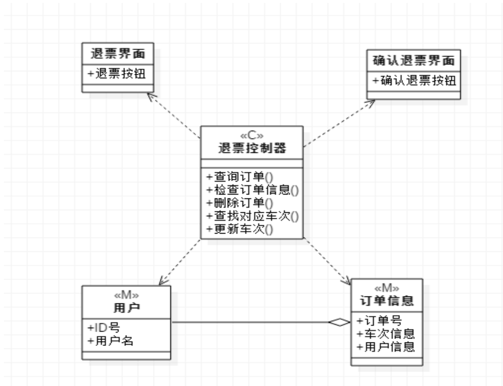
图 7 退票类图
