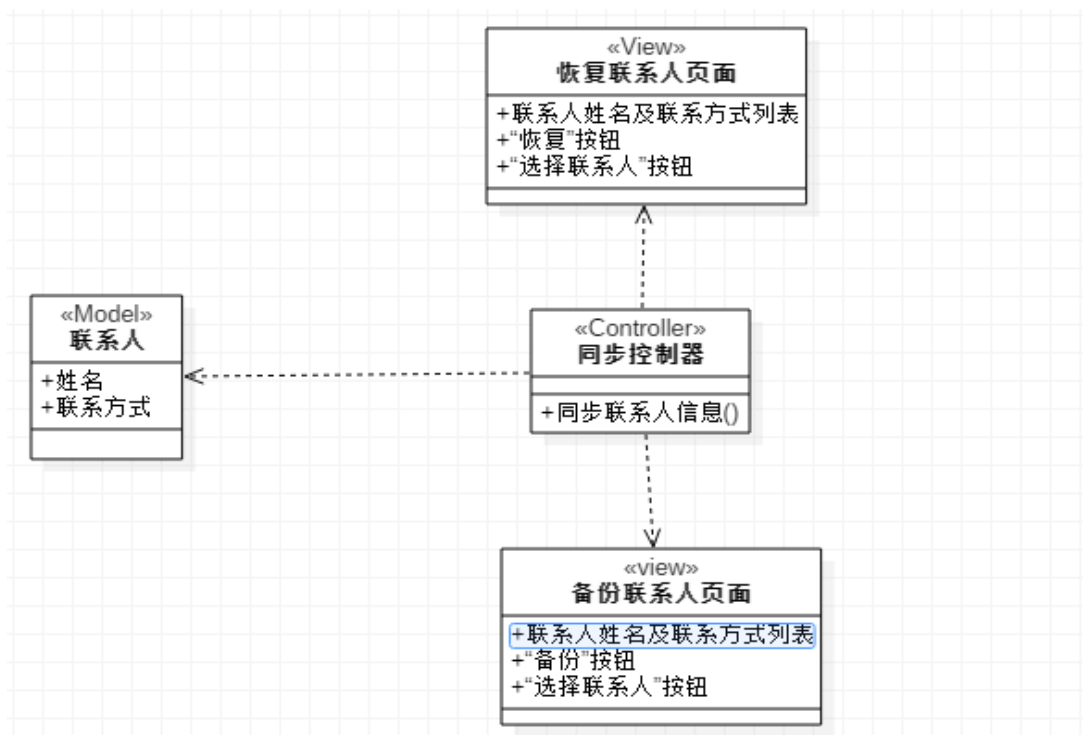
图 4：同步联系人类型图
