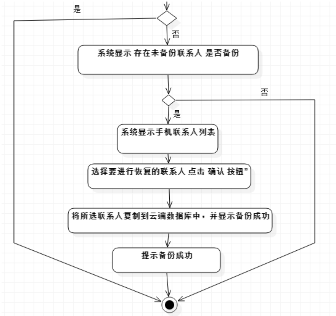
图 2：同步联系人活动图
