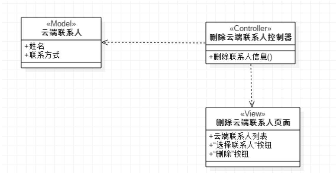
图 5：管理云端联系人图
