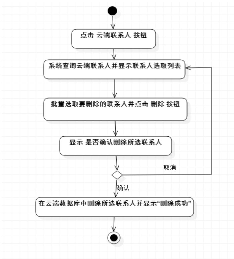
图 3：管理云端联系人活动图
