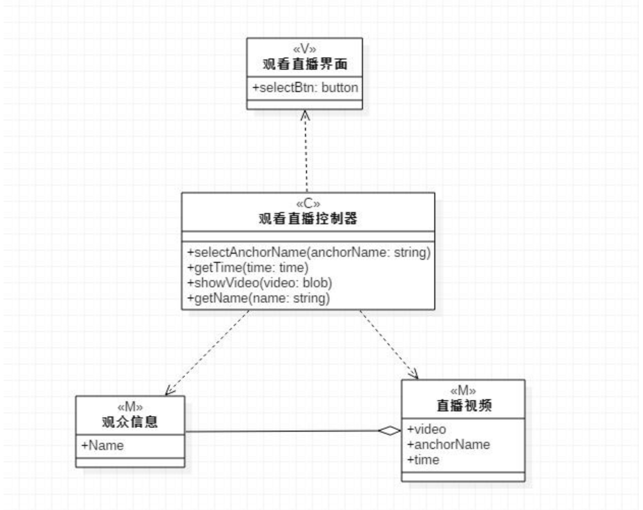
观众打赏主播类模型
