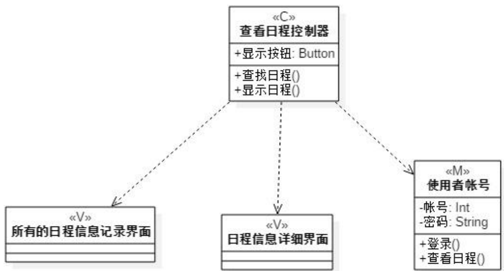
图 3-1: 创建日程-类图
