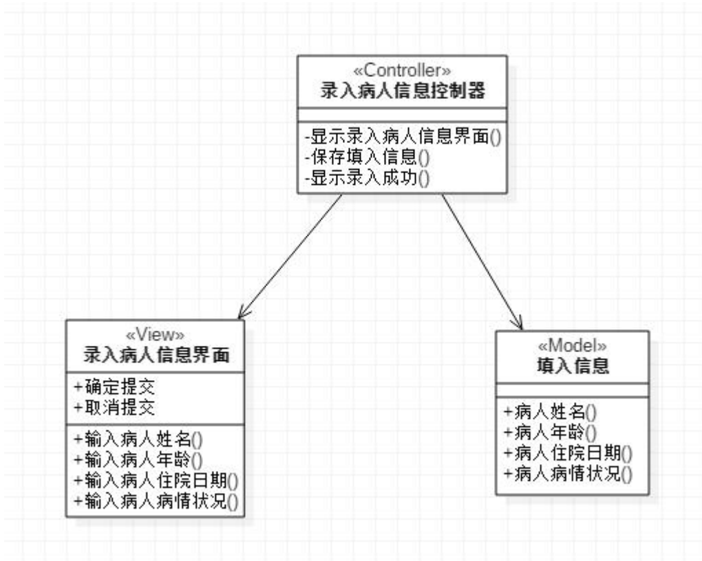
图 4：录入病人的临床医疗信息类图
