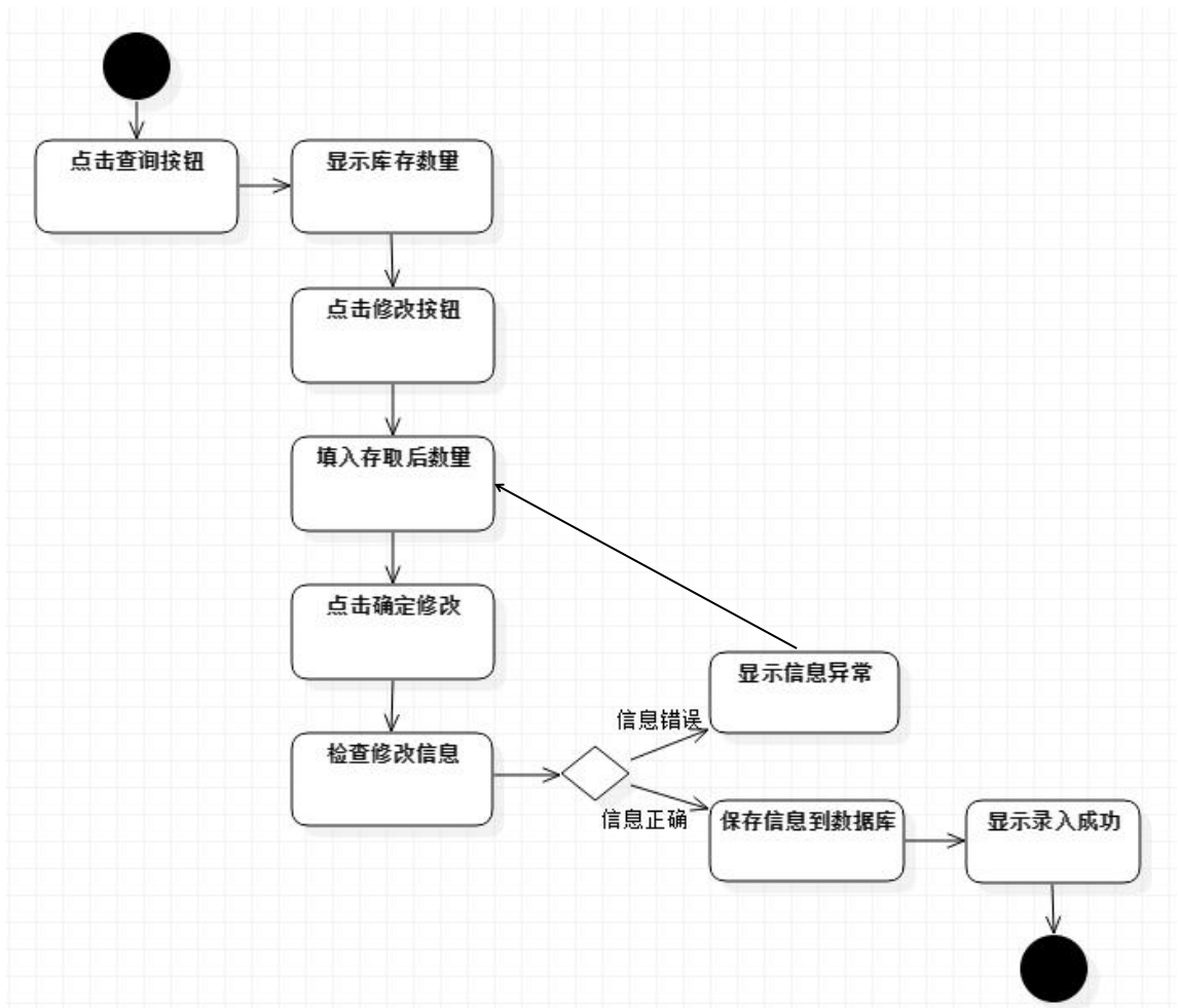
图 3：修改药房药品库存活动图
