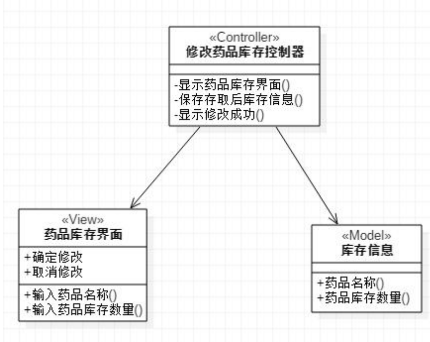
图 5：修改药房药品库存
