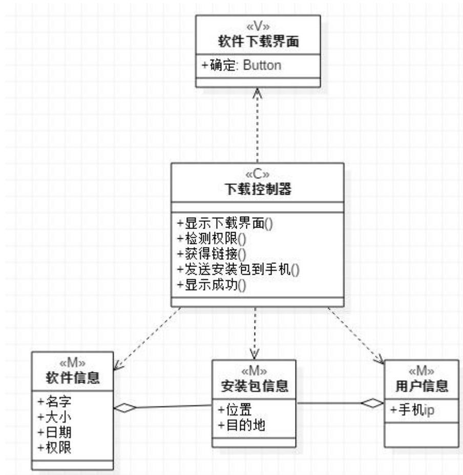
图 5. 下载类建模
