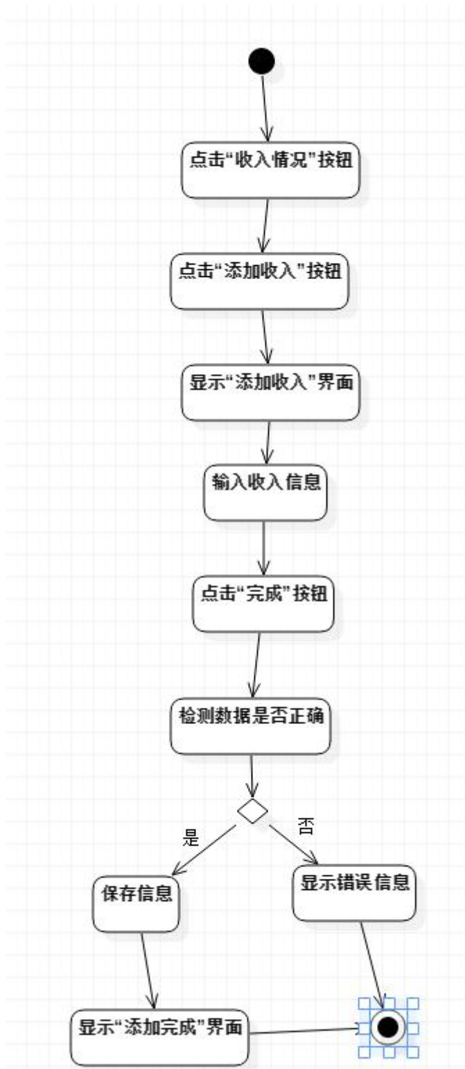
录入收入情况活动图
