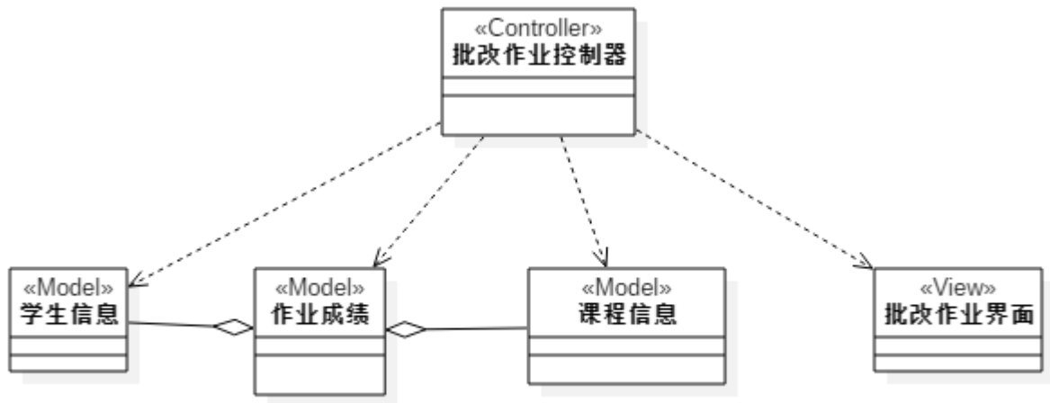
图 5：“记录作业成绩”类图
