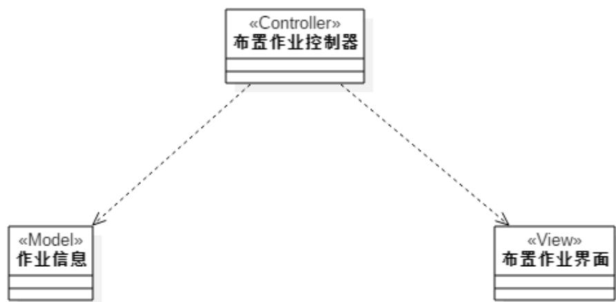
图 4：“布置作业任务”类图
