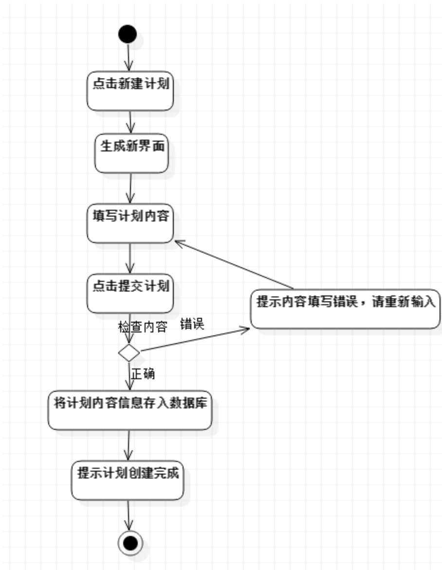
图 2: U001 活动图
