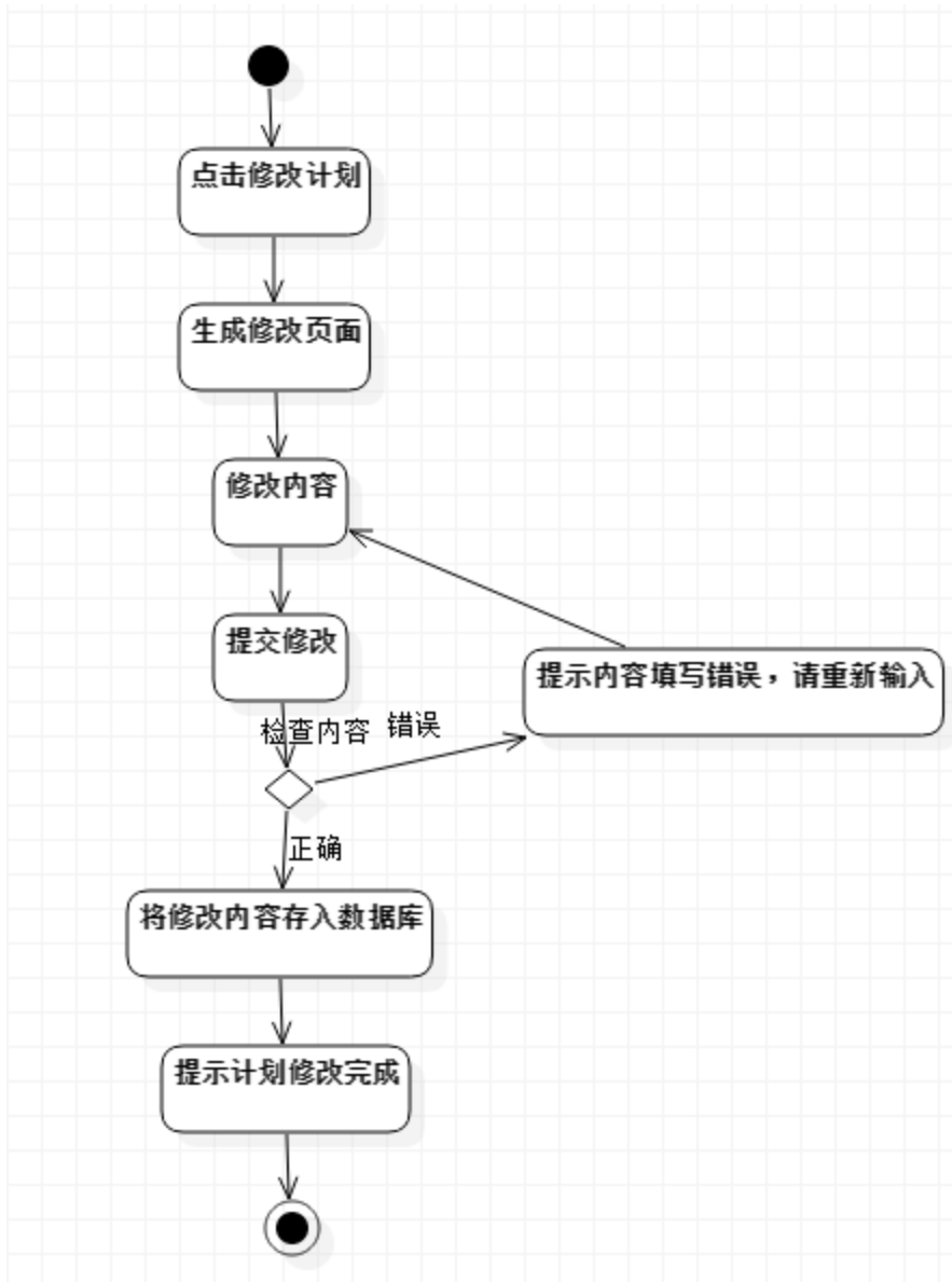
图 3: U002 活动图
