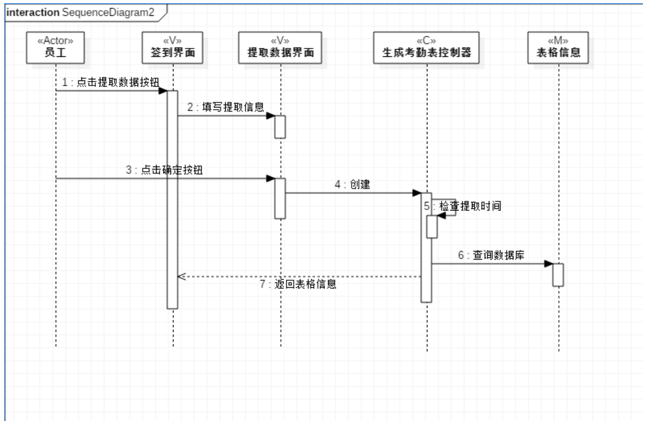
图 7：生成考勤表的顺序模型
