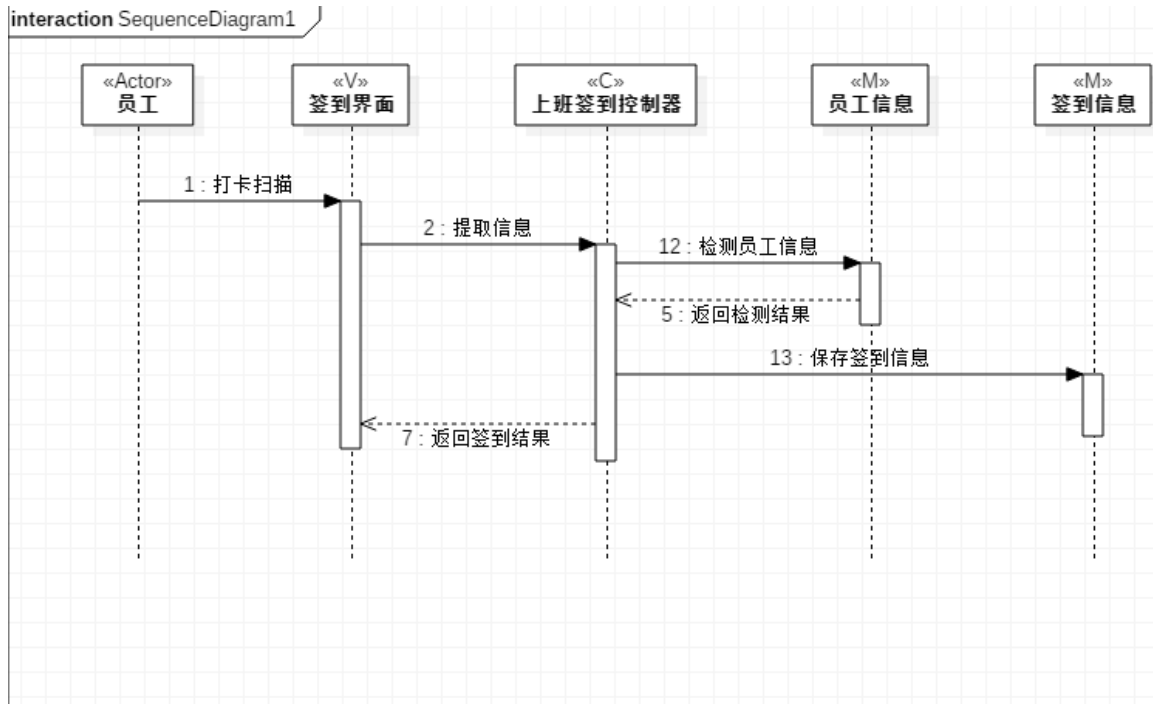
图 6：上班签到的顺序模型
