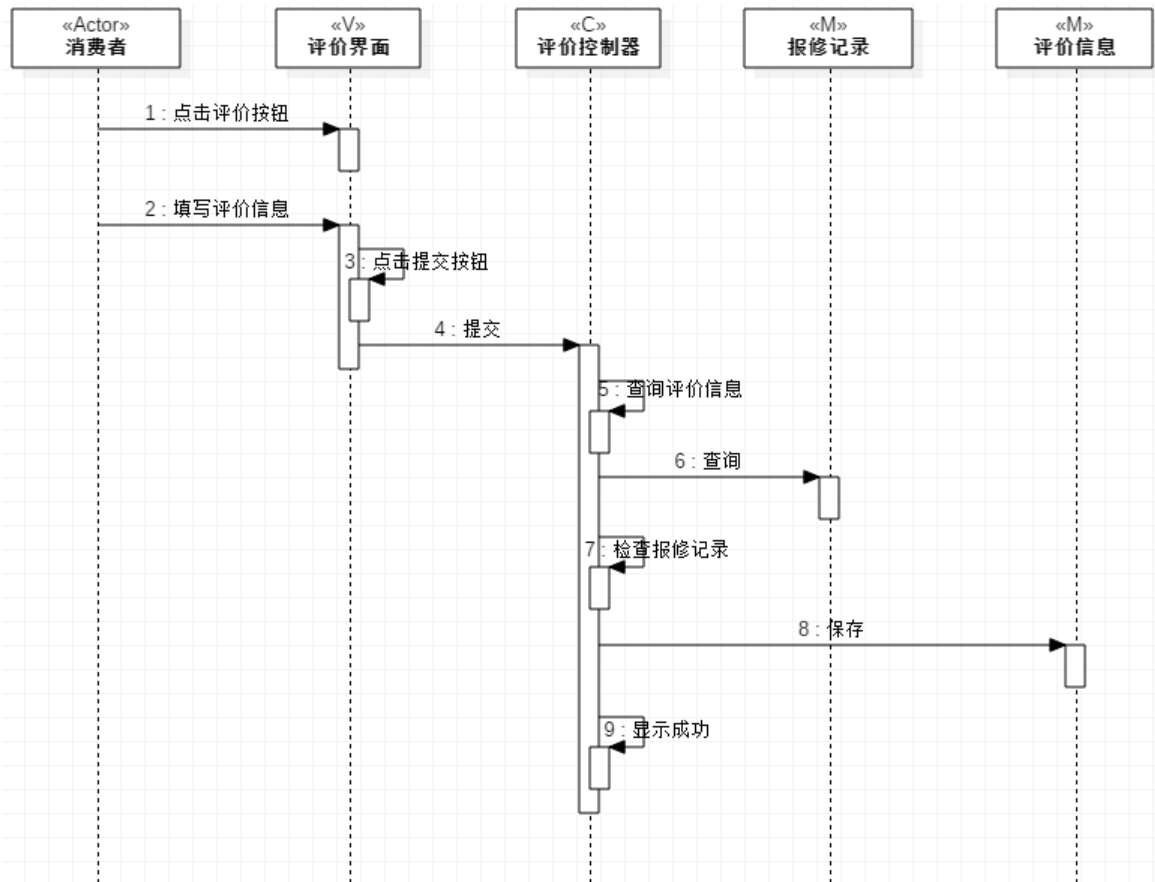
图 7 评价顺序图
