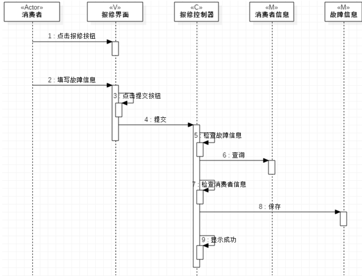
图 6 报修顺序图
