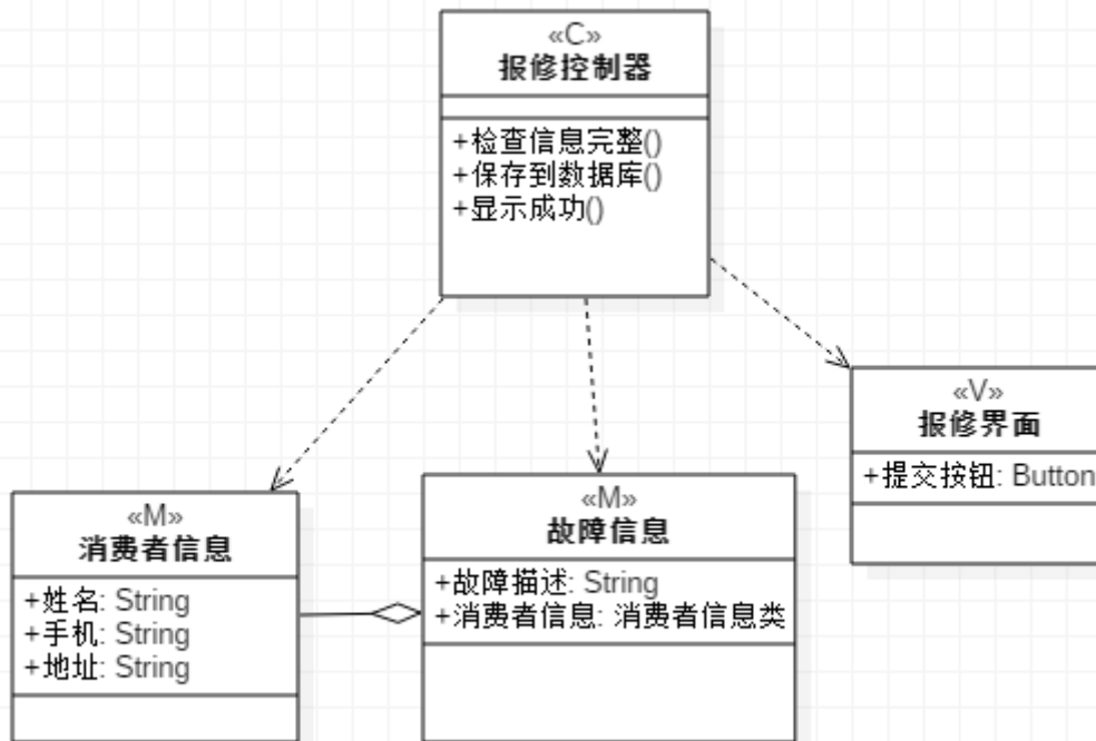
图 4 报修类图
