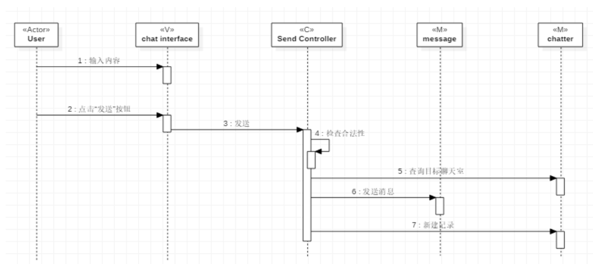
图 7: 发送消息顺序图
