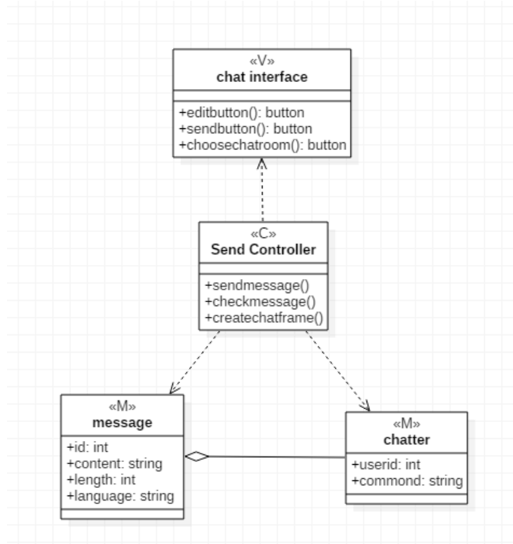
图 5：发送消息类图
