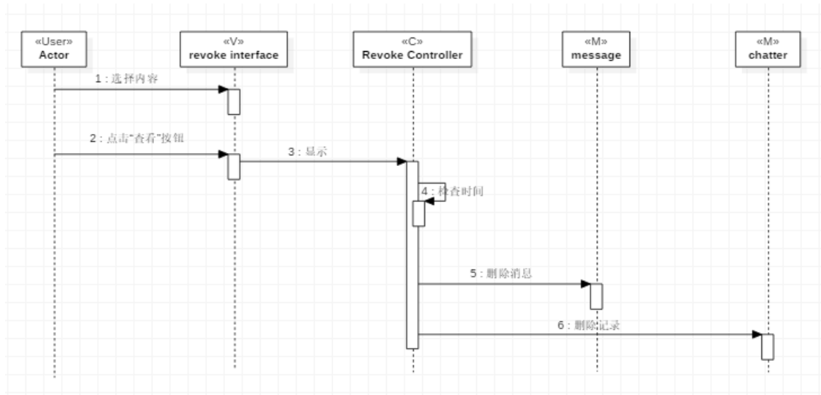
图 7: 撤回消息顺序图
