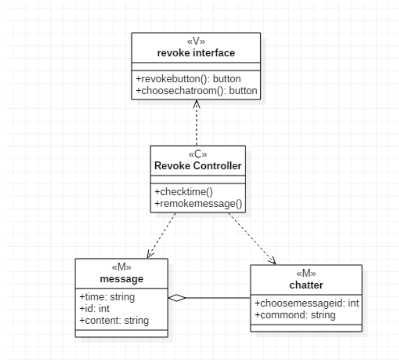
图 6：撤回消息类图
