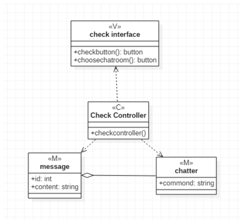
图 6: 查看历史消息类图
