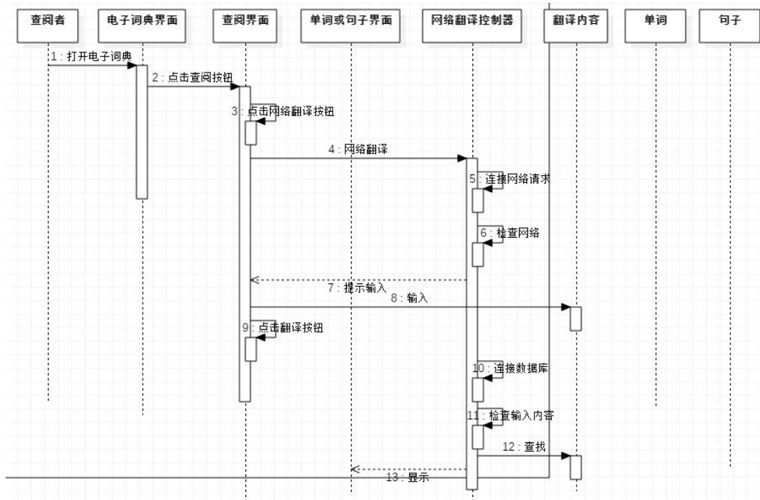
图 3：网络翻译顺序图
