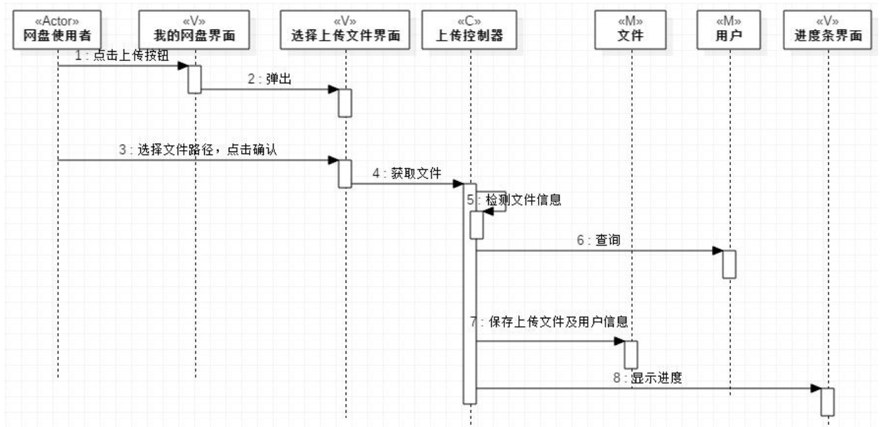
图 6：上传文件顺序图
