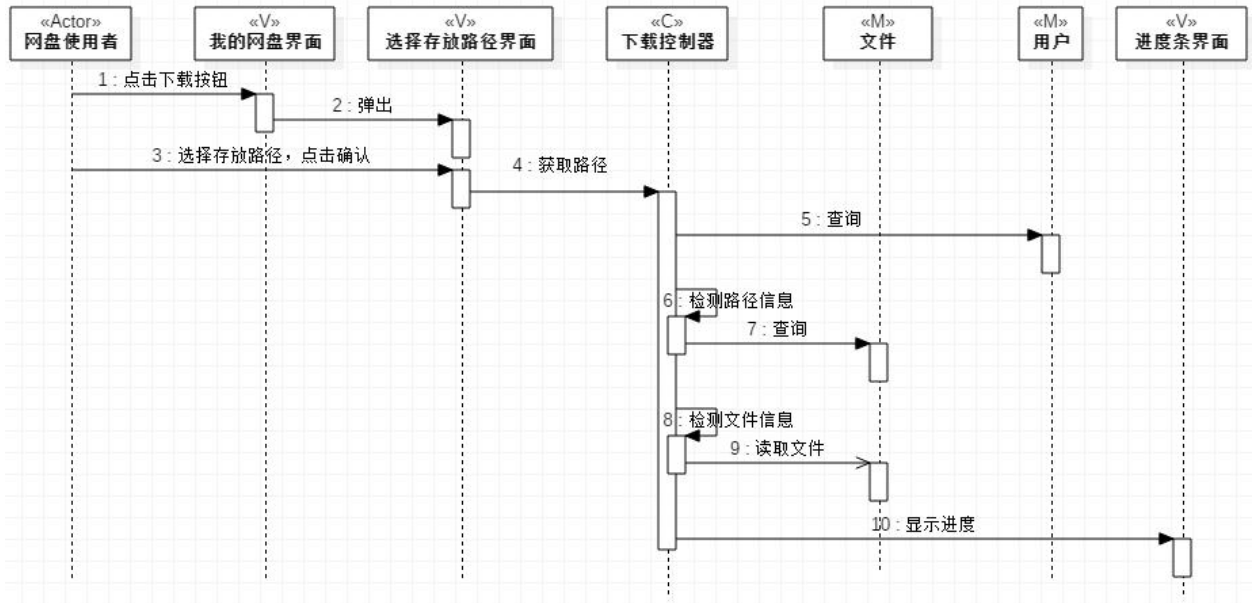
图 5：下载文件顺序图
