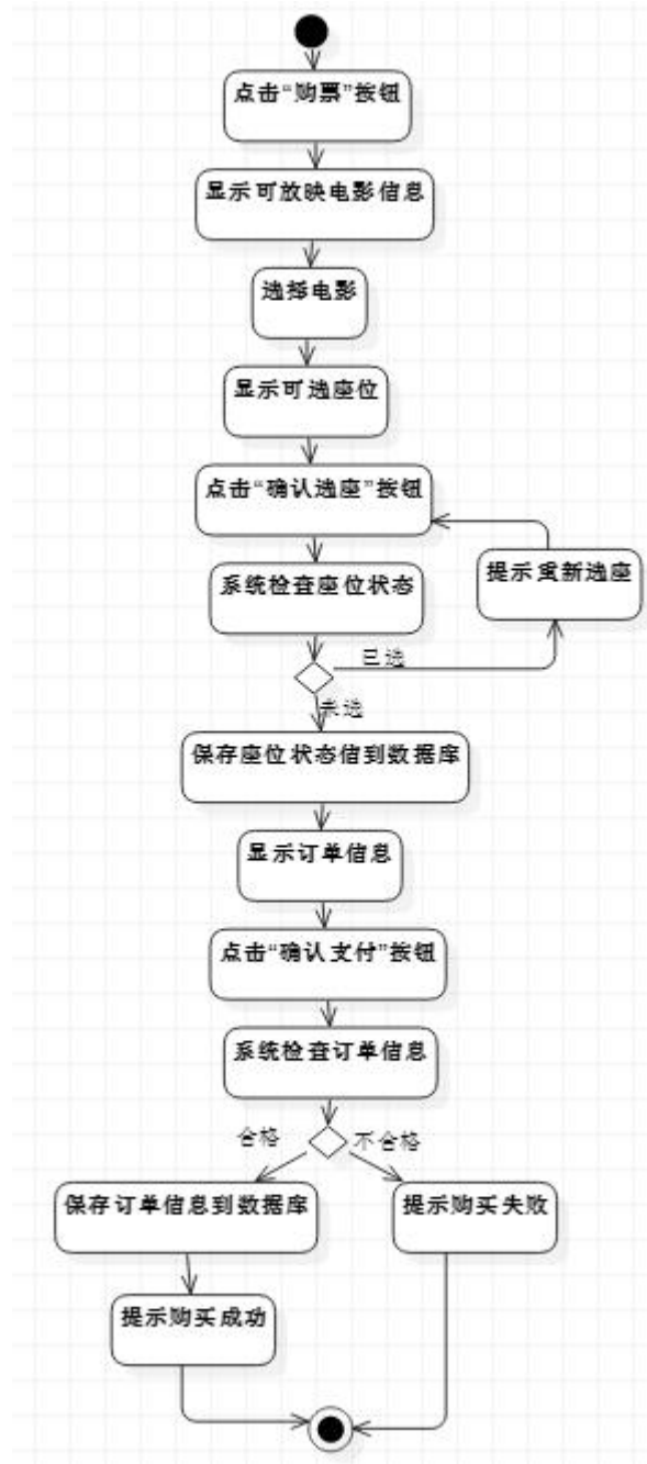
用例“订购电影票”活动图
