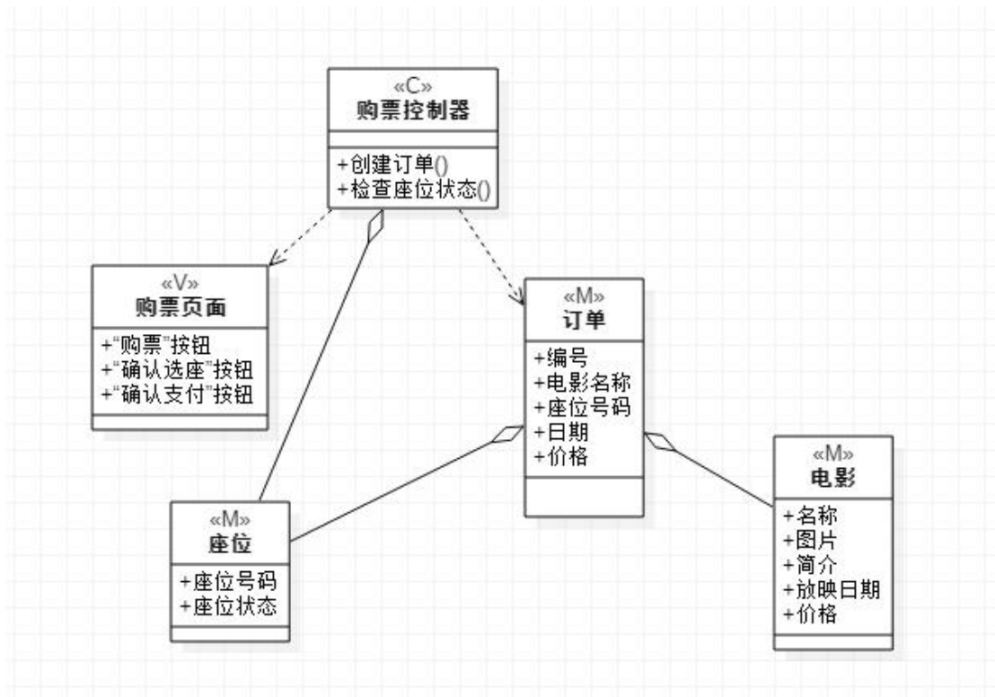
“订购电影票”类图
