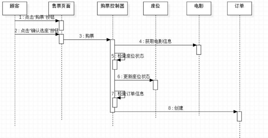
订购电影票”时序图
