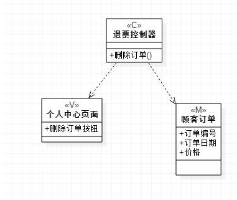
“退电影票”类图
