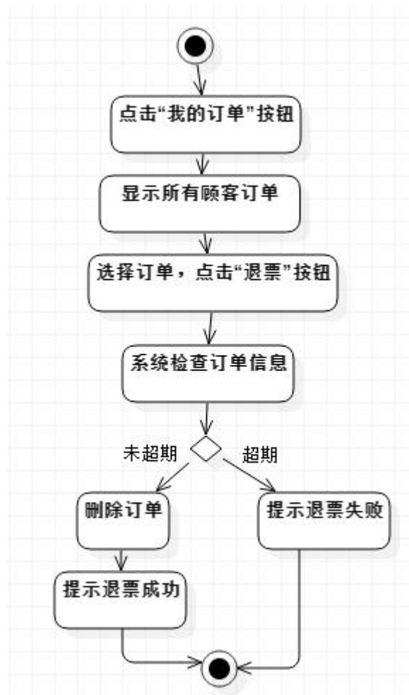
用例“退电影票”活动图
