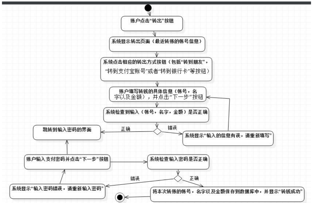
图 1:转账活动图
