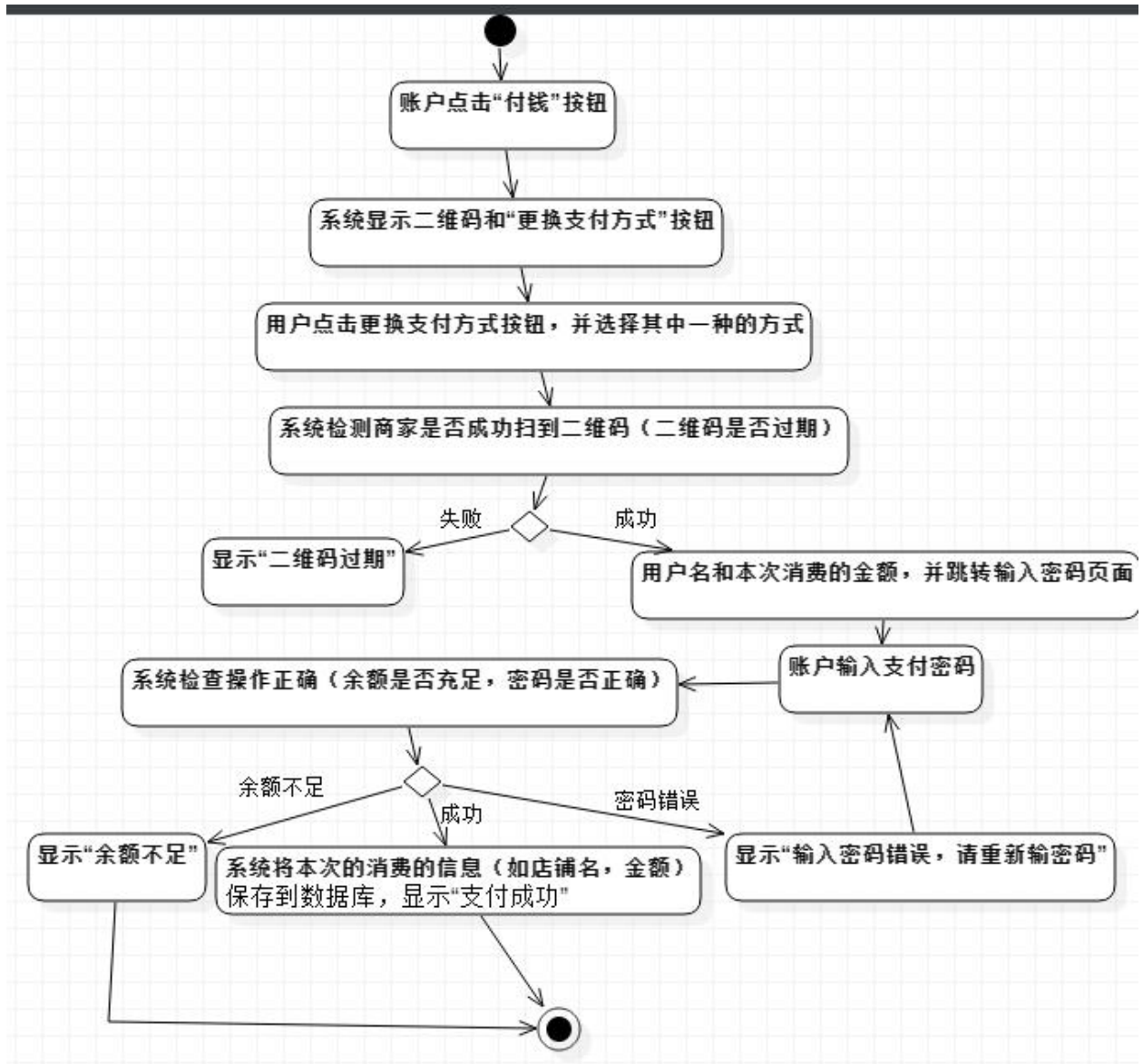
图 2:活动图
