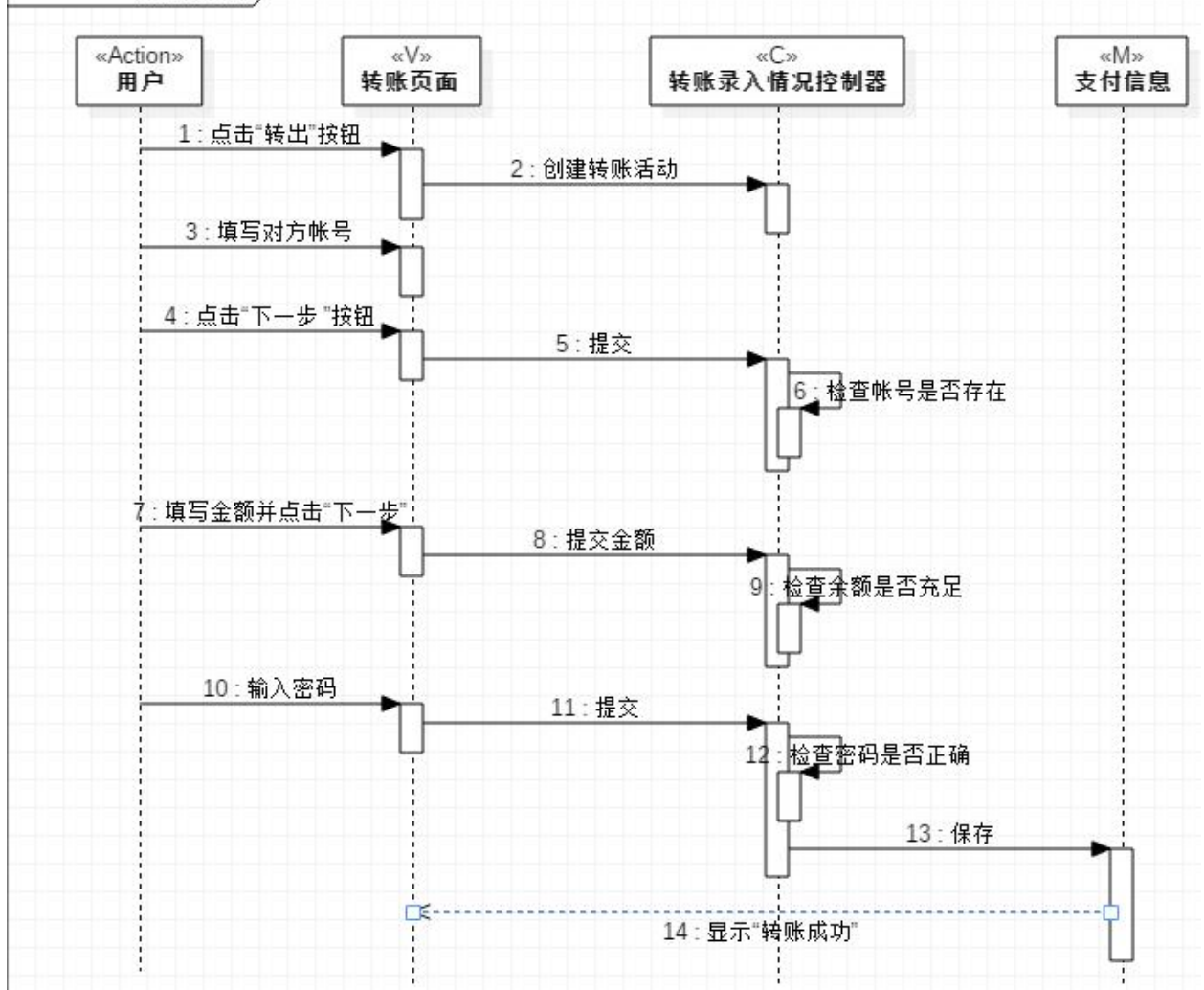
图 5: 转账顺序图
