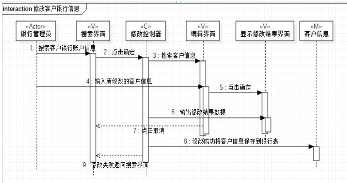
修改客户银行账户顺序模型图
