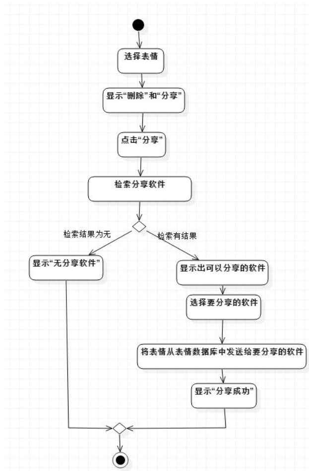
用例 UC003 分享表情活动图
