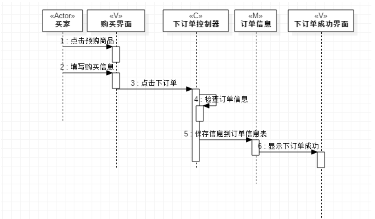
图 7：下订单顺序图
