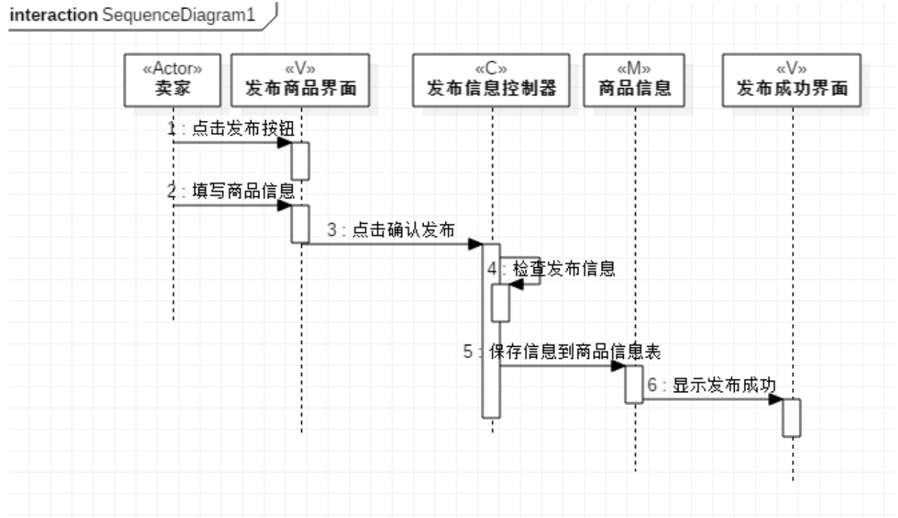
图 6：发布信息顺序图
