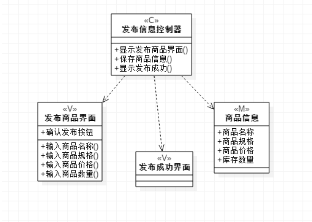
图 4：发布信息类图
