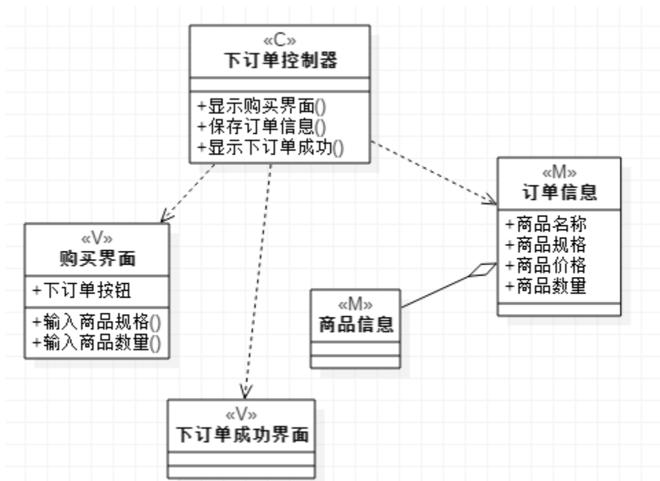
图 5：下订单类图
