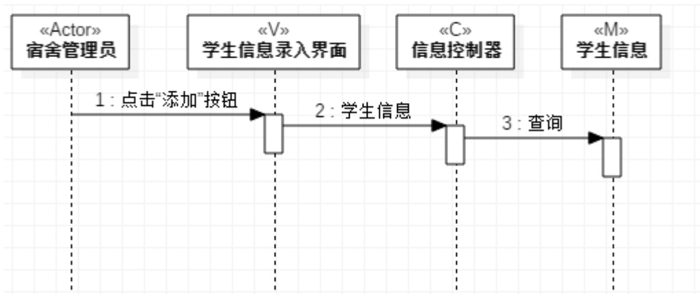
图 6: 录入学生信息顺序图
