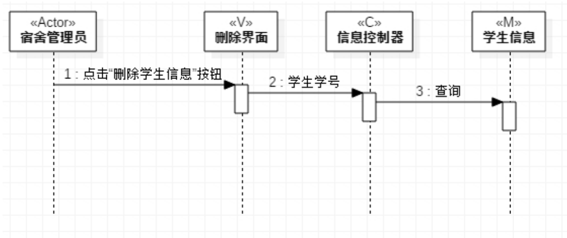
图 7: 删除学生信息控制器
