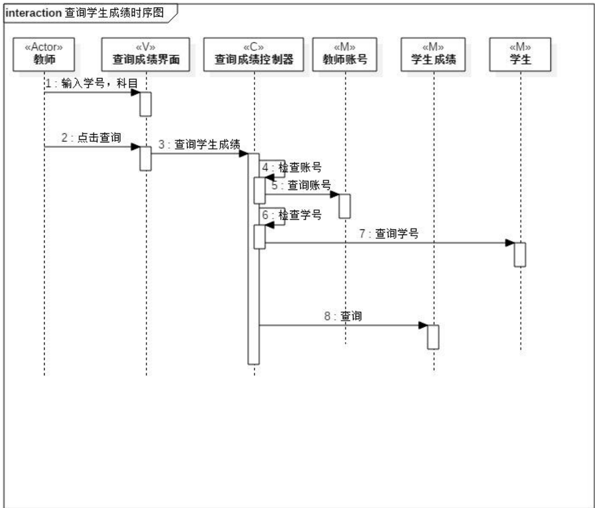
图 9: 查询学生成绩时序图
