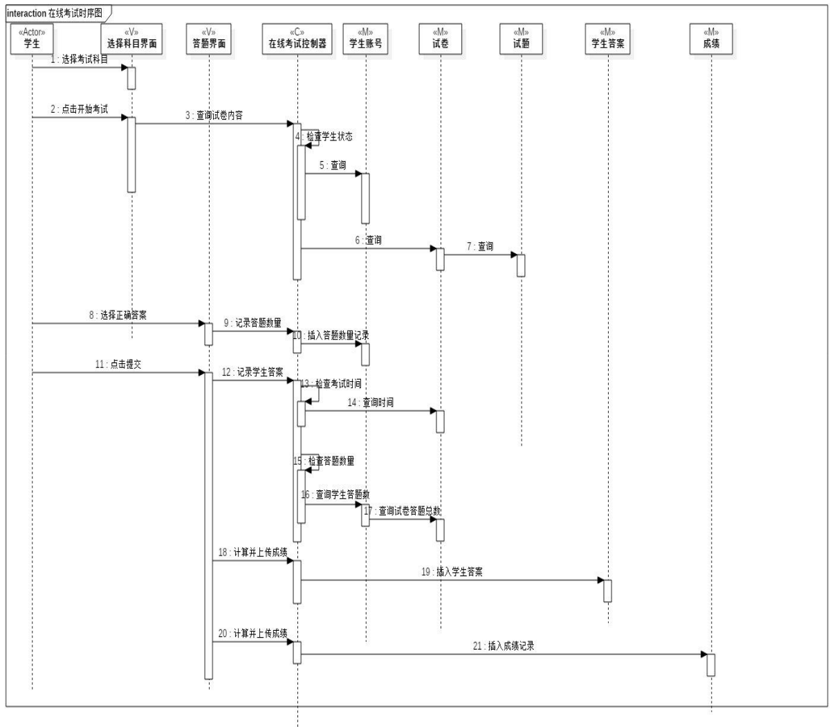
图 10: 在线考试时序图
