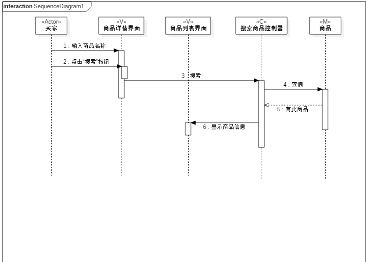
图 7：搜索商品顺序图
