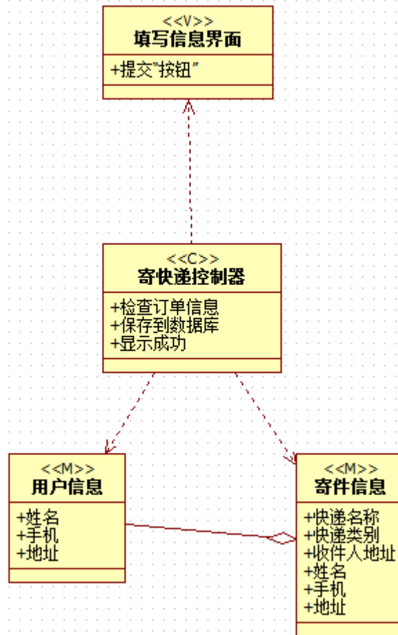
图 4：寄件类图
