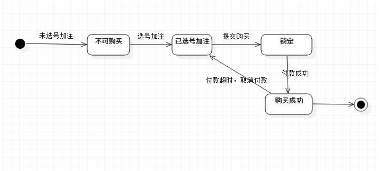
订单状态转换图
