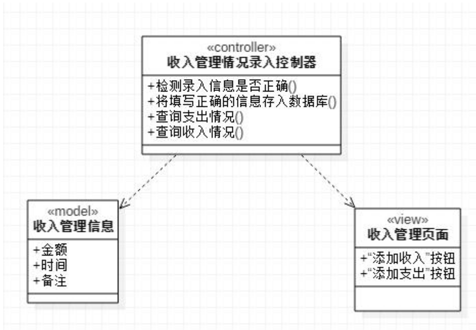
收支管理系统类图
