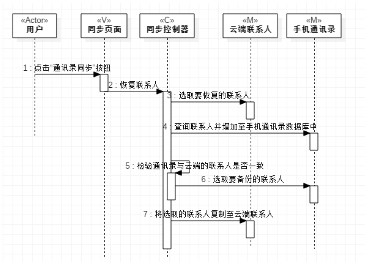
图 6：同步联系人顺序图
