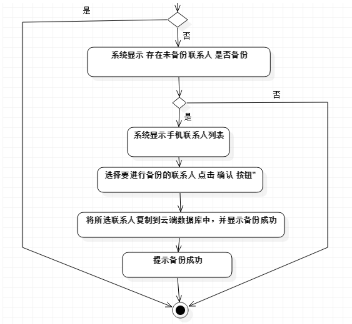
图 2: 同步联系人活动图<2>
