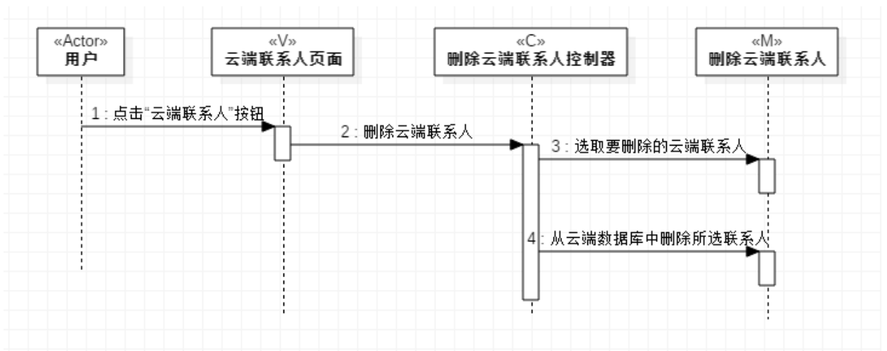
图 7：删除云端联系人顺序图
