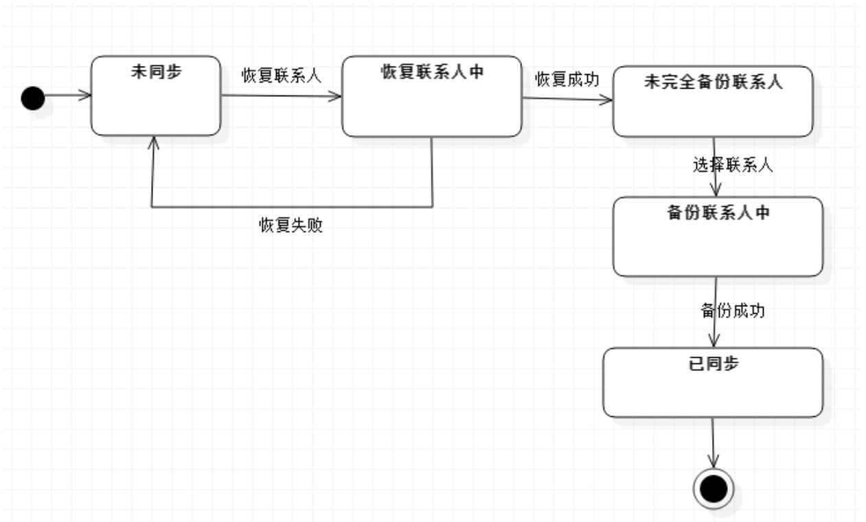
图 8：联系人同步状态图
