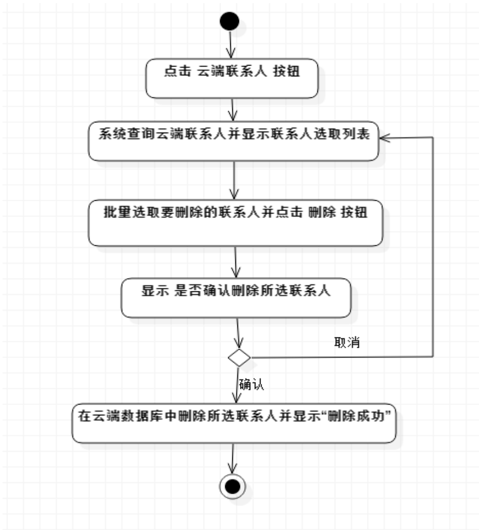
图 3：删除云端联系人活动图
