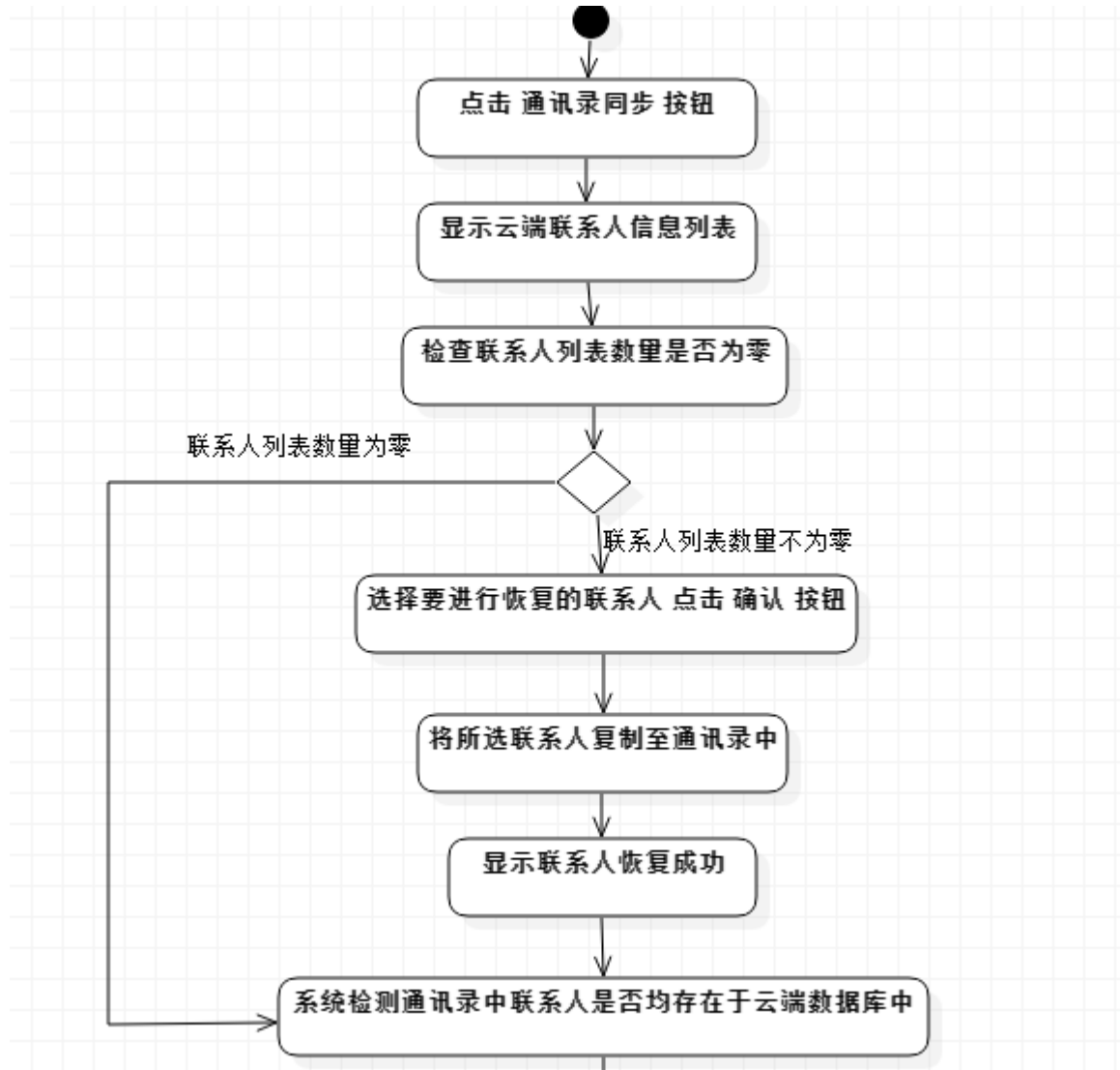
图 2：同步联系人活动图<1>
