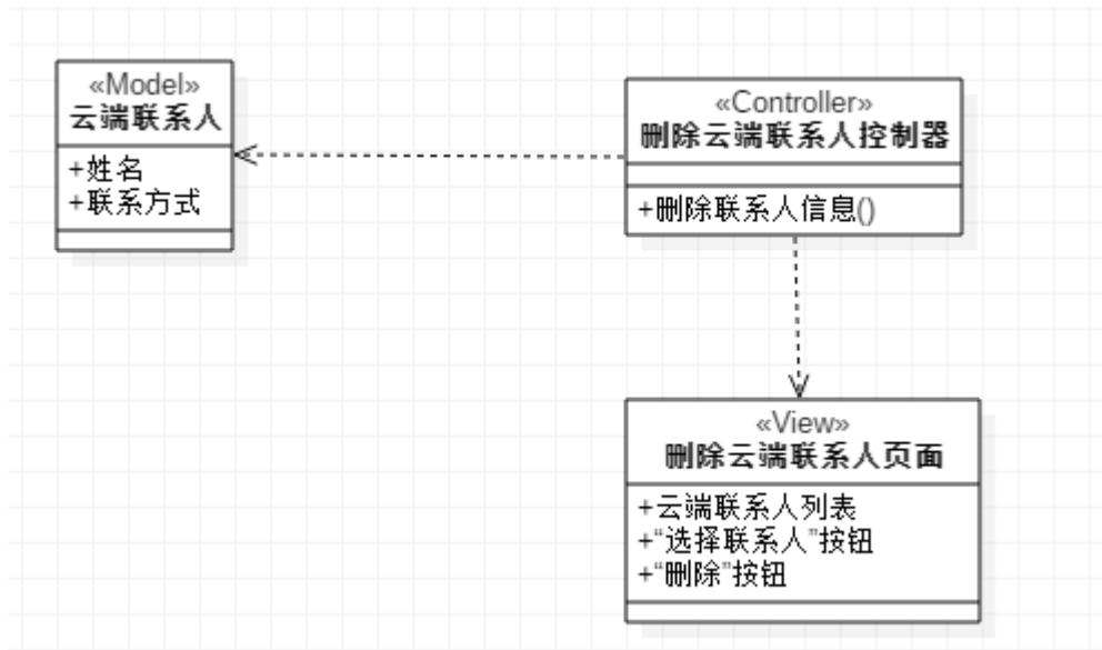
图 5：删除云端联系人类图
