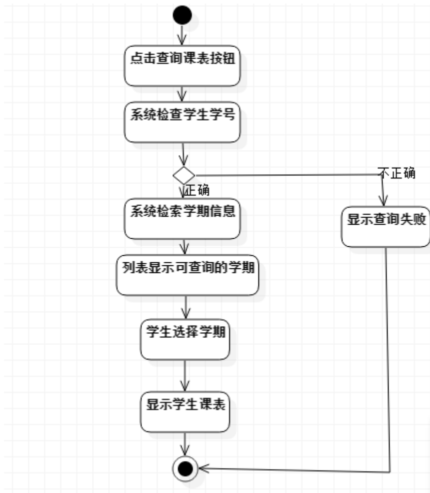
图 2：查询个人课表活动图
