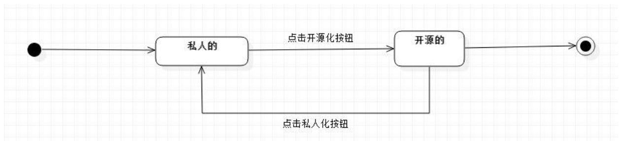
仓库状态图
