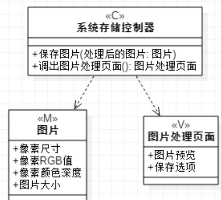
UC002 类图：
