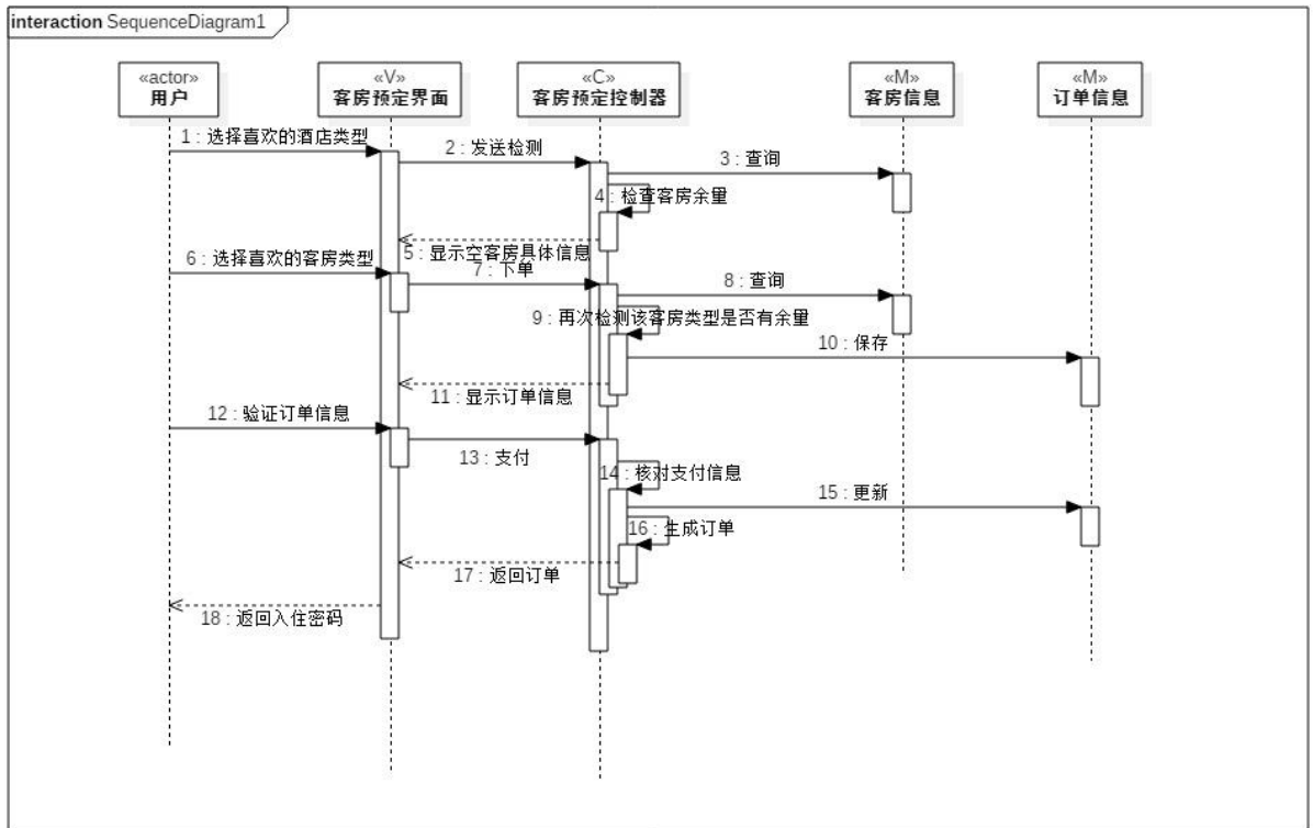
图 4-1：酒店客房预订顺序图
