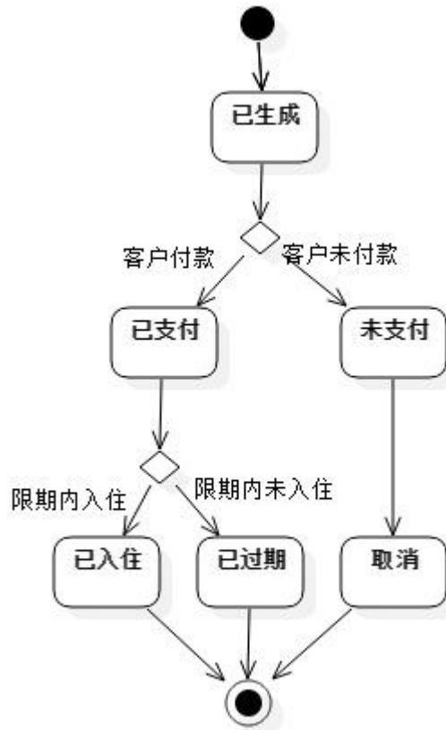
图 5-1: 客房信息状态图
