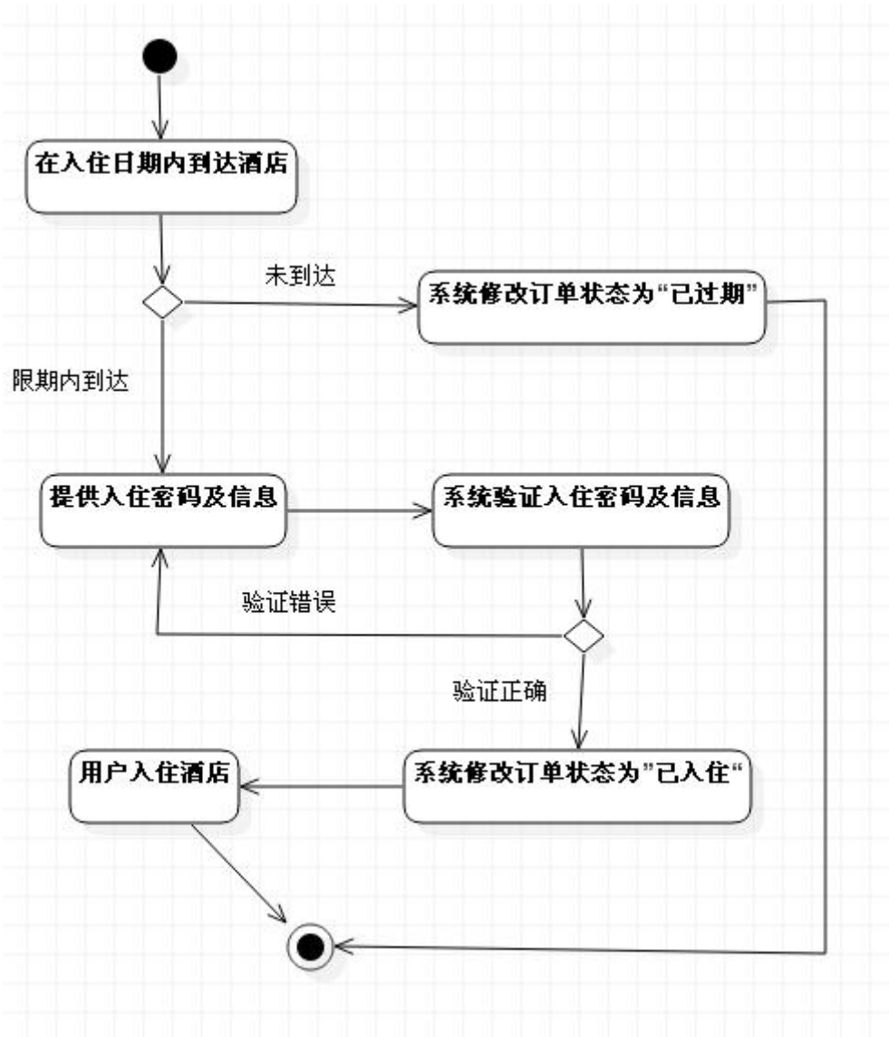
图 2-2：酒店客房入住系统用例图
