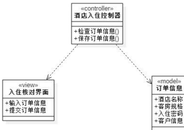
图 3-1：酒店客房预订类图
