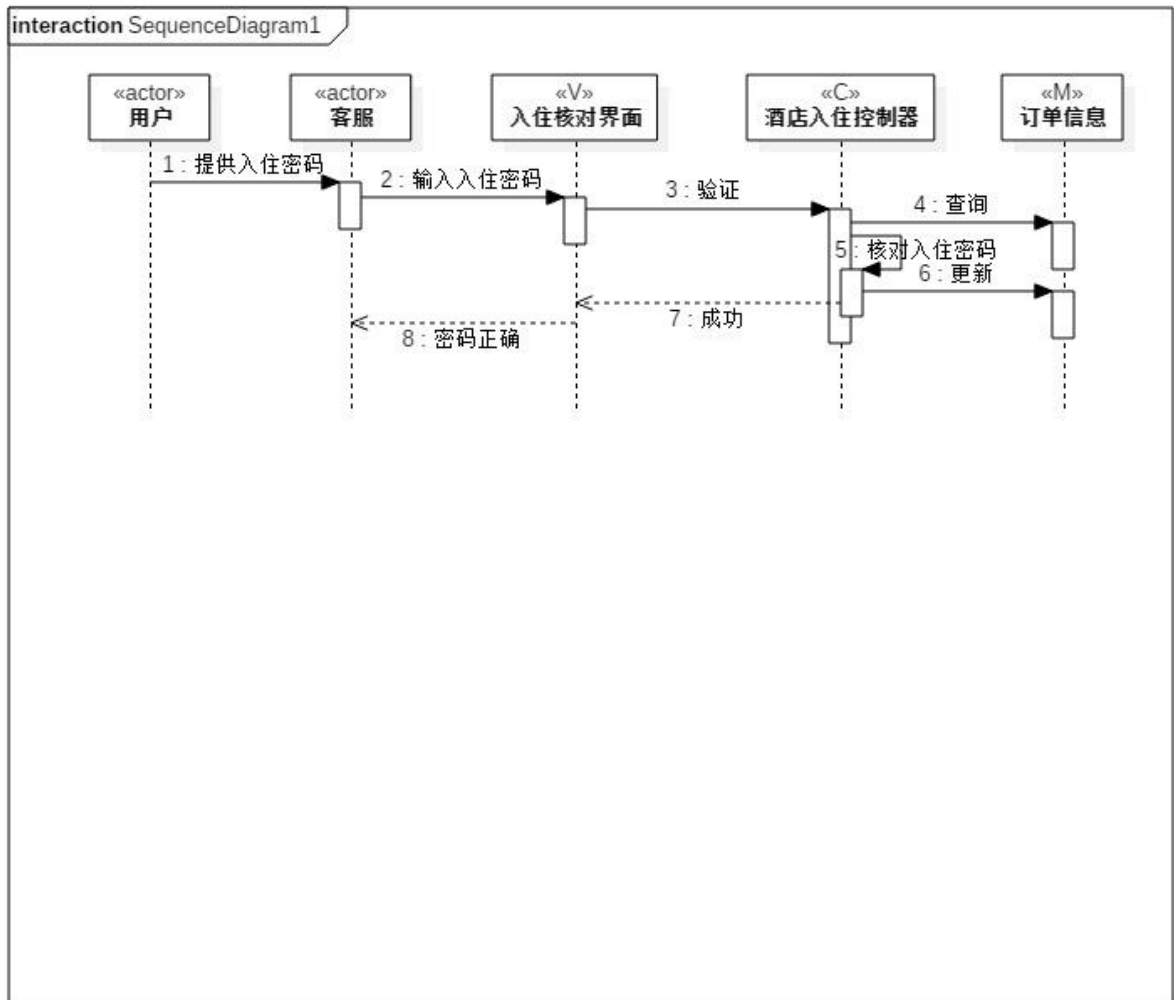
图 4-2: 酒店客房入住顺序图
