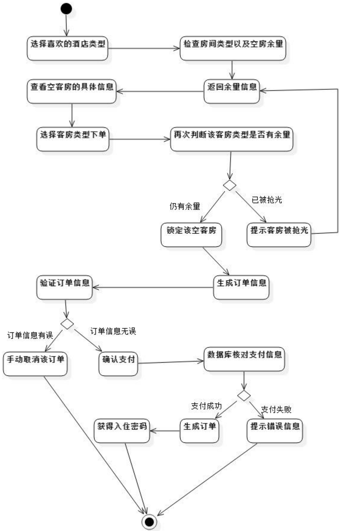
图 2-1：酒店客房预定系统活动图
