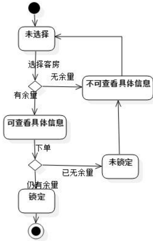
图 5-1: 客房信息状态图
