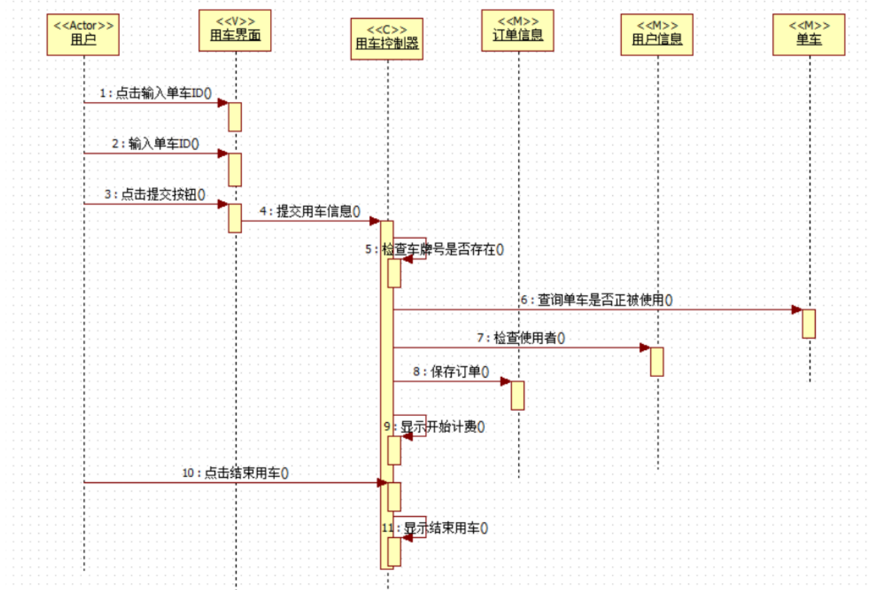
用车顺序图
