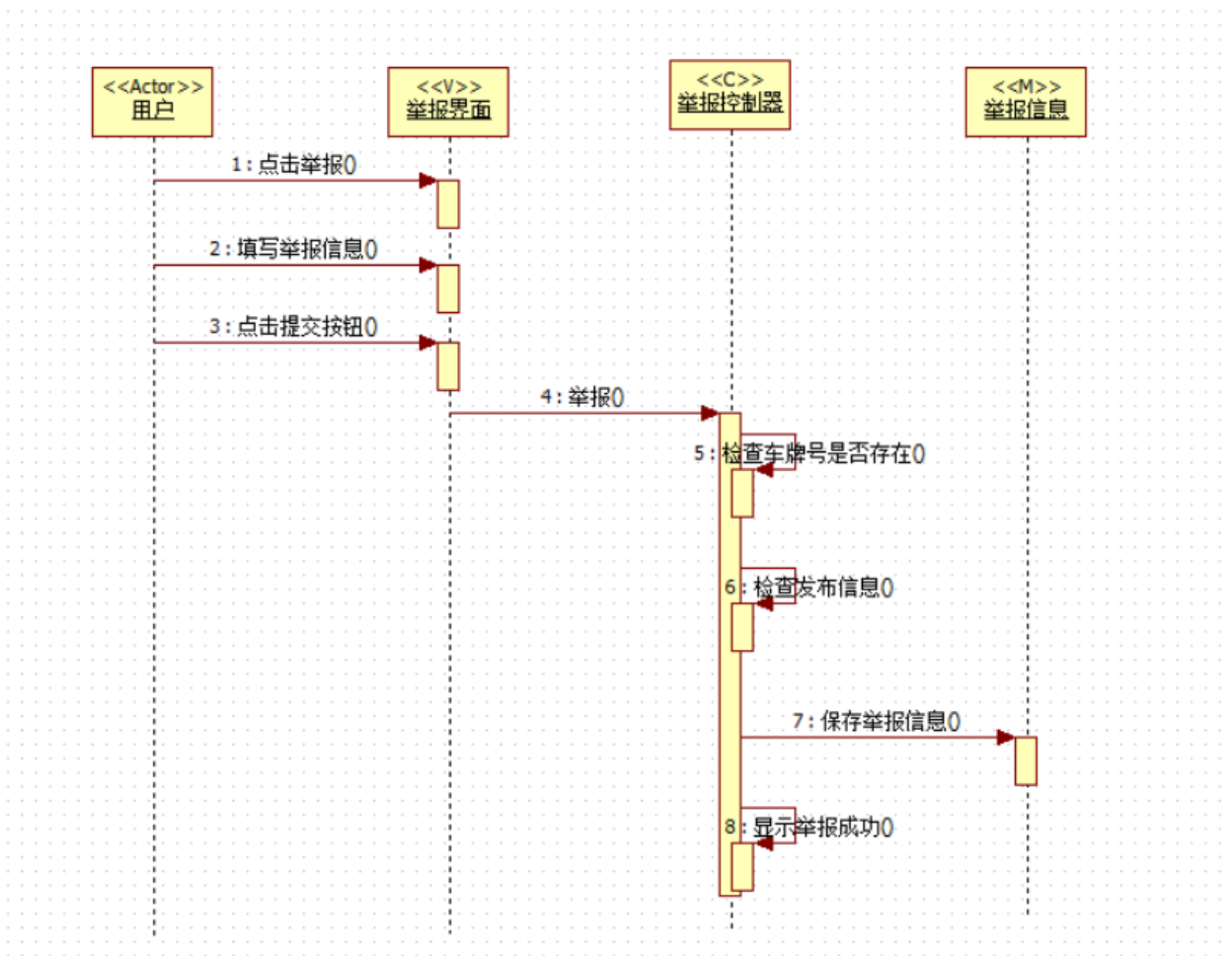
举报顺序图
