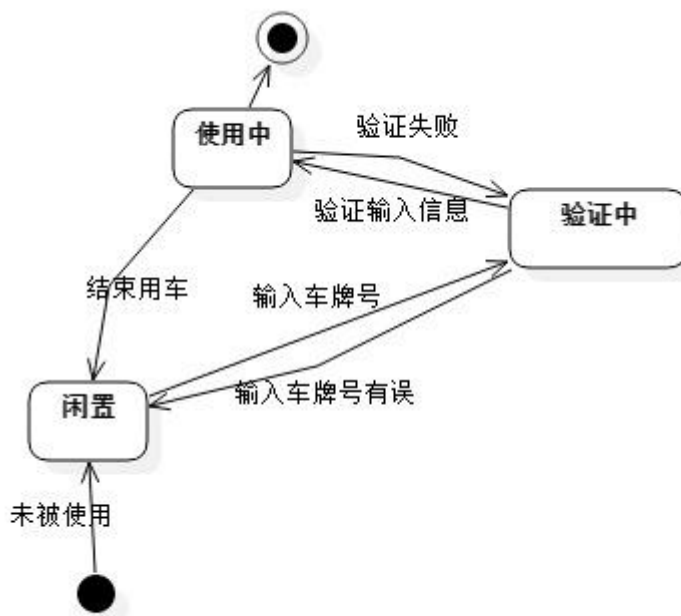
单车状态图
