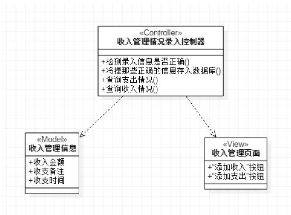
收支管理系统类图
