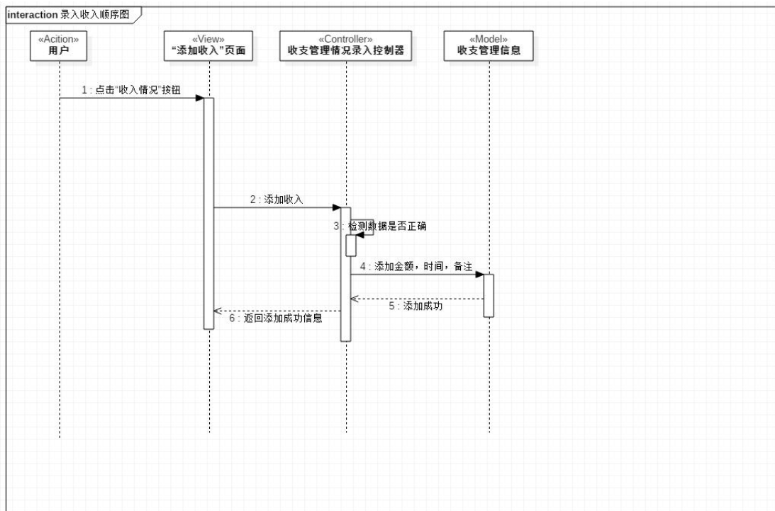
录入收入顺序图
