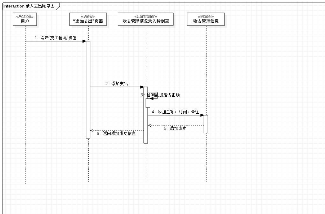
录入支出顺序图
