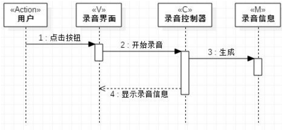
图 10: 录音顺序图
