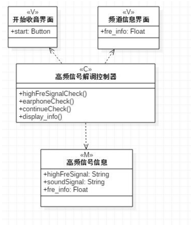
图 5: 收音类图
