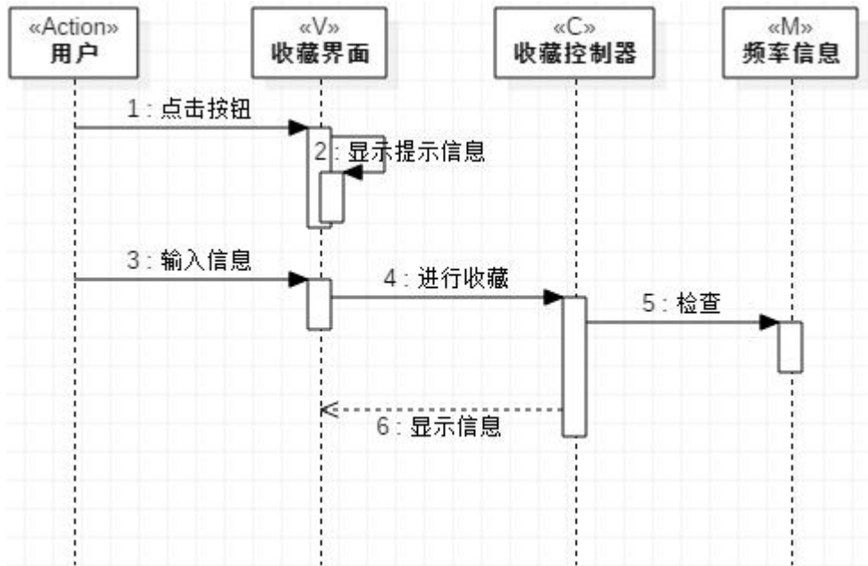
图 9: 收藏顺序图
