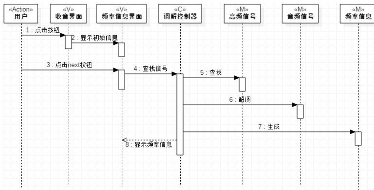
图 8: 收音顺序图
