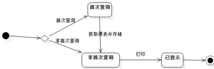
状态图：课表信息状态图
