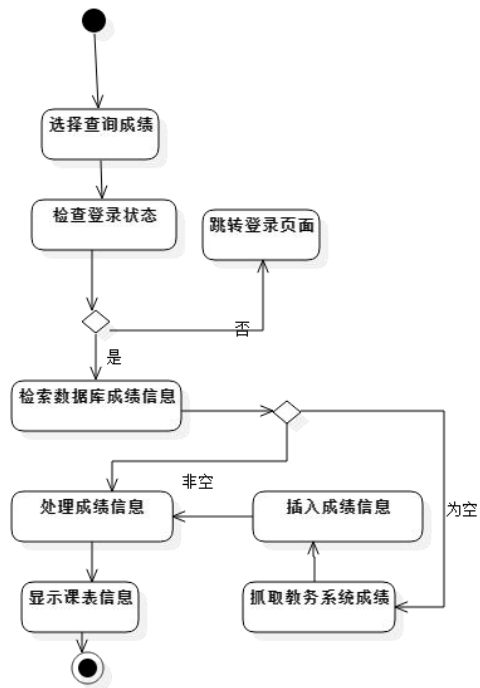
图 2：UC002 查询成绩活动图
