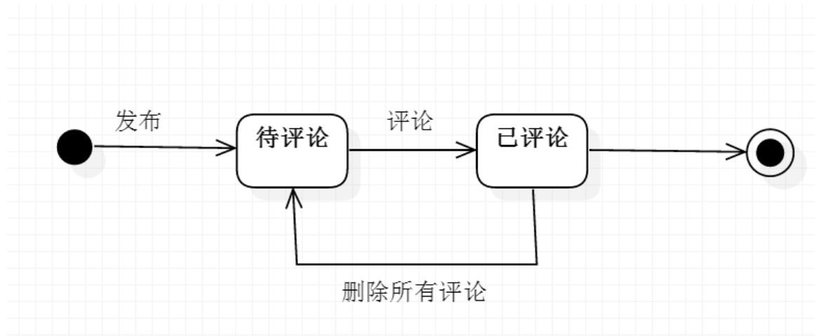
图 5-1 “文字动态信息” 状态图
