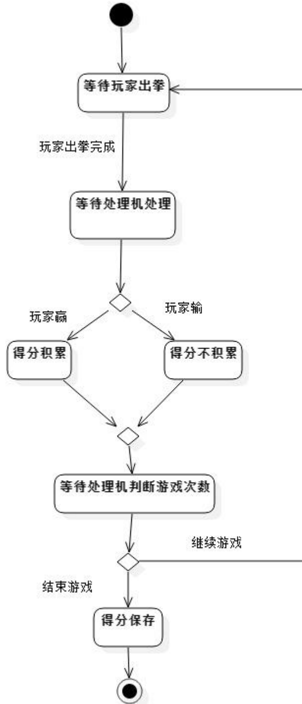
图 8：“游戏”状态图
