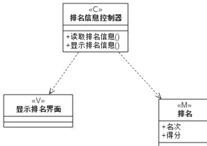
图 5:排名类图
