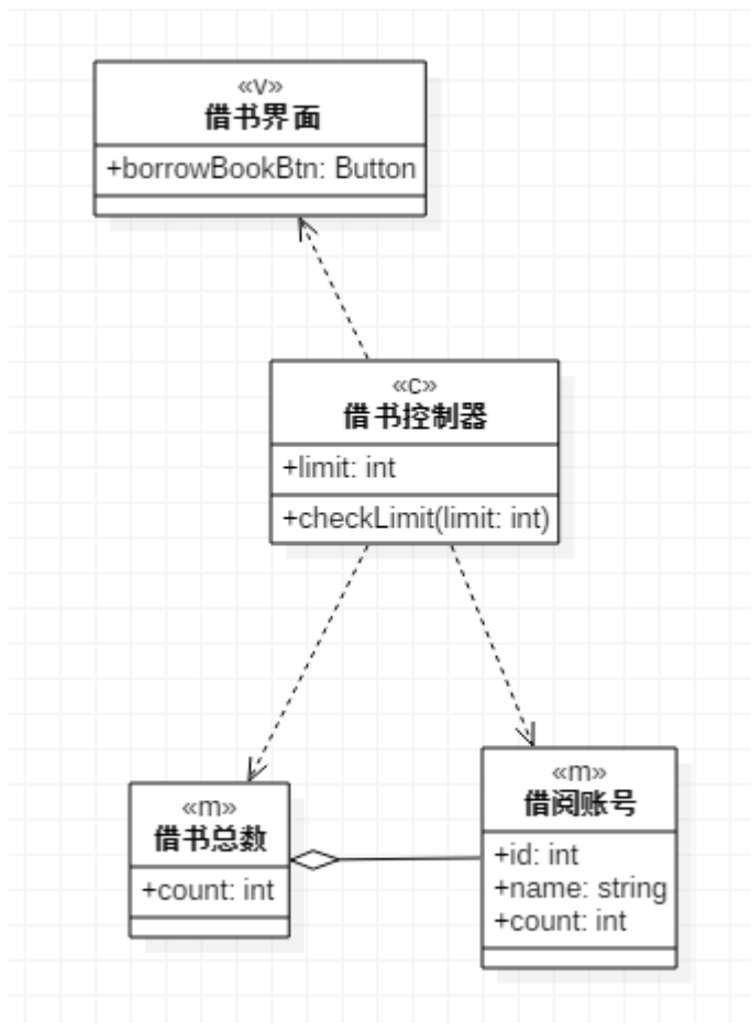
UC002 的类图:
