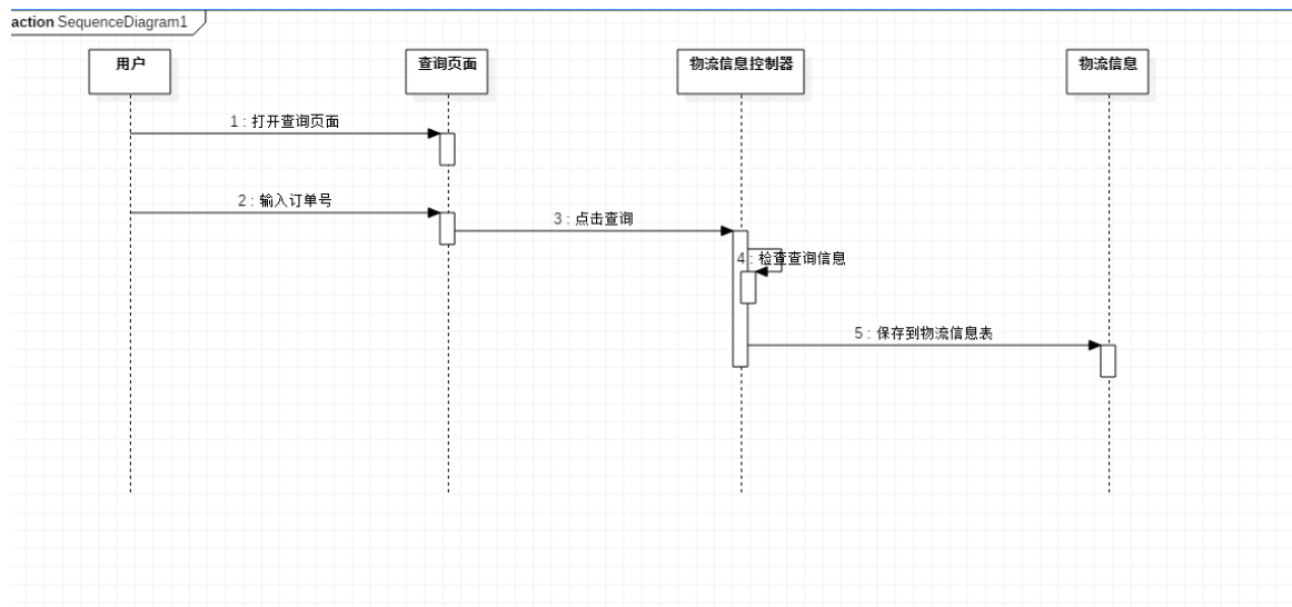
图 7: 查询顺序图
