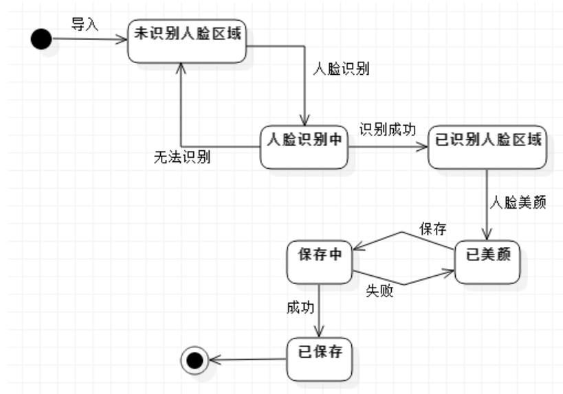
“图片” 状态图
