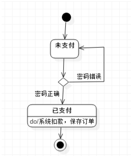
订单的状态图
