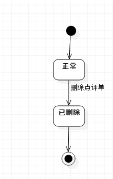
点评单的状态图
