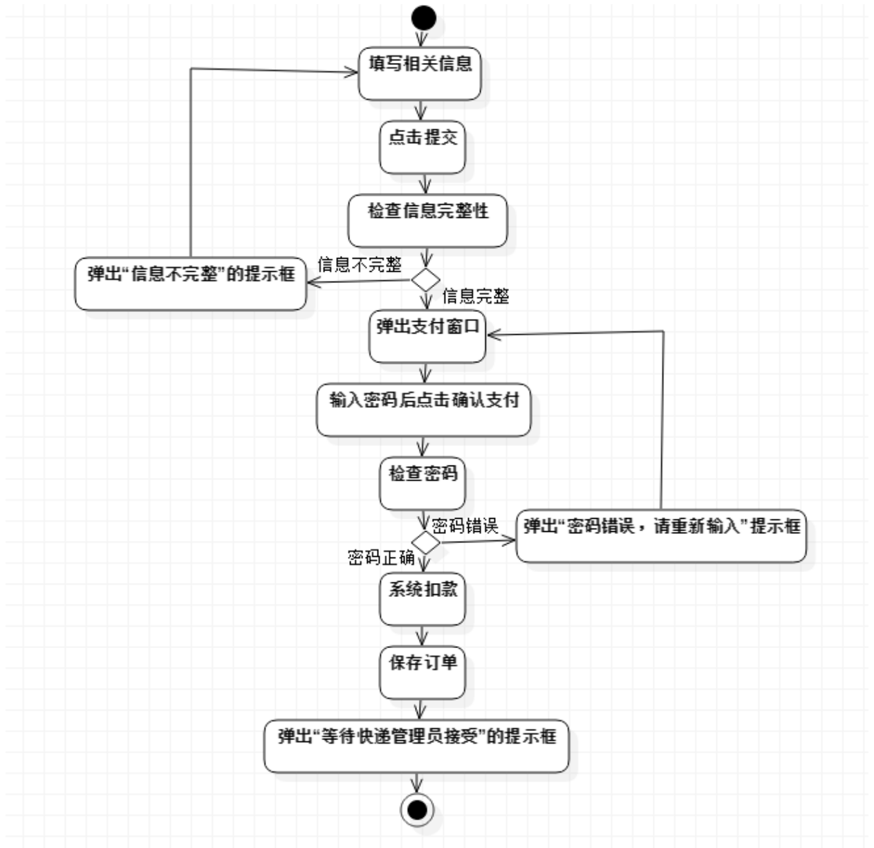
发布代收快递请求的活动图
