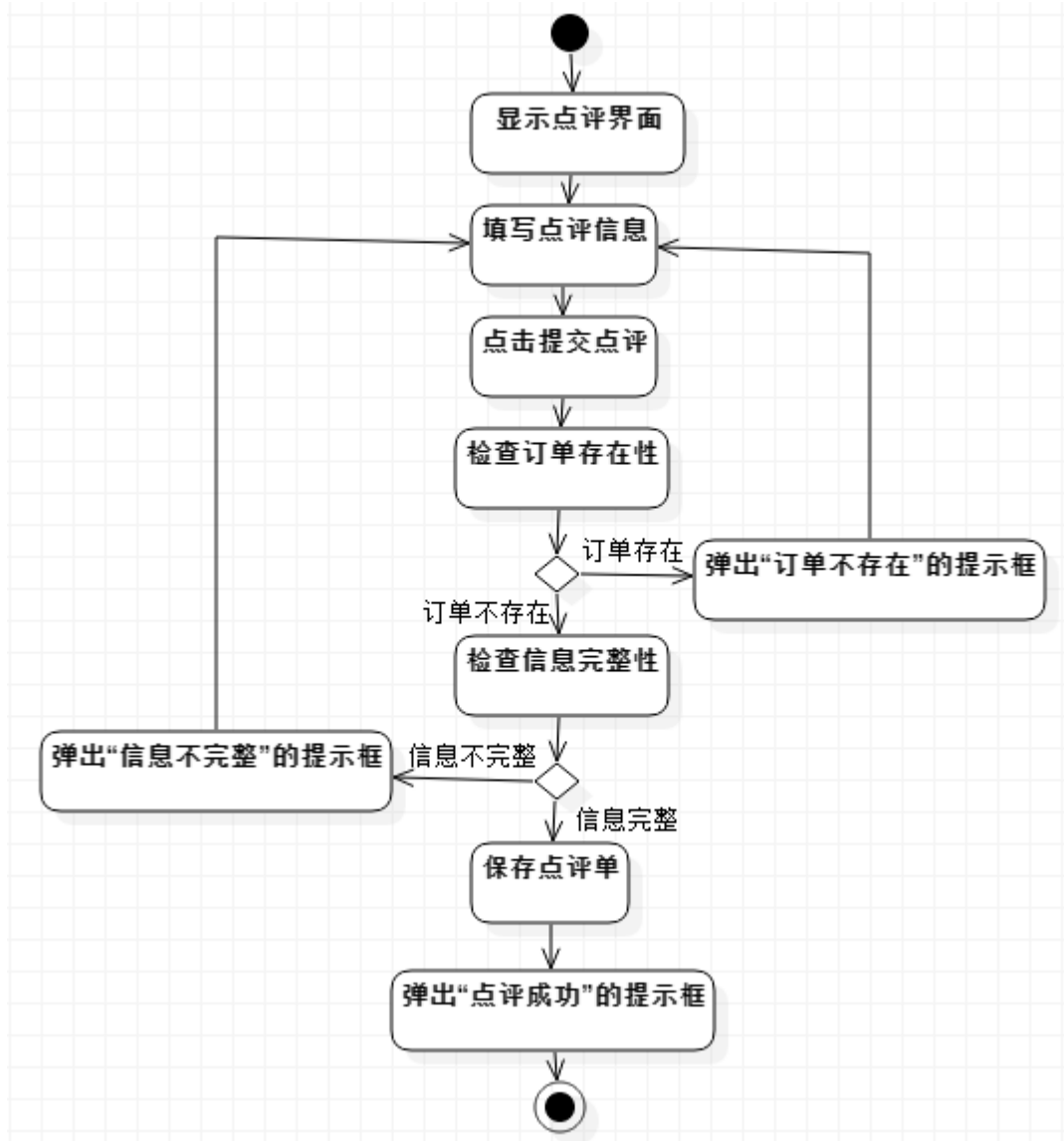
点评订单的活动图
