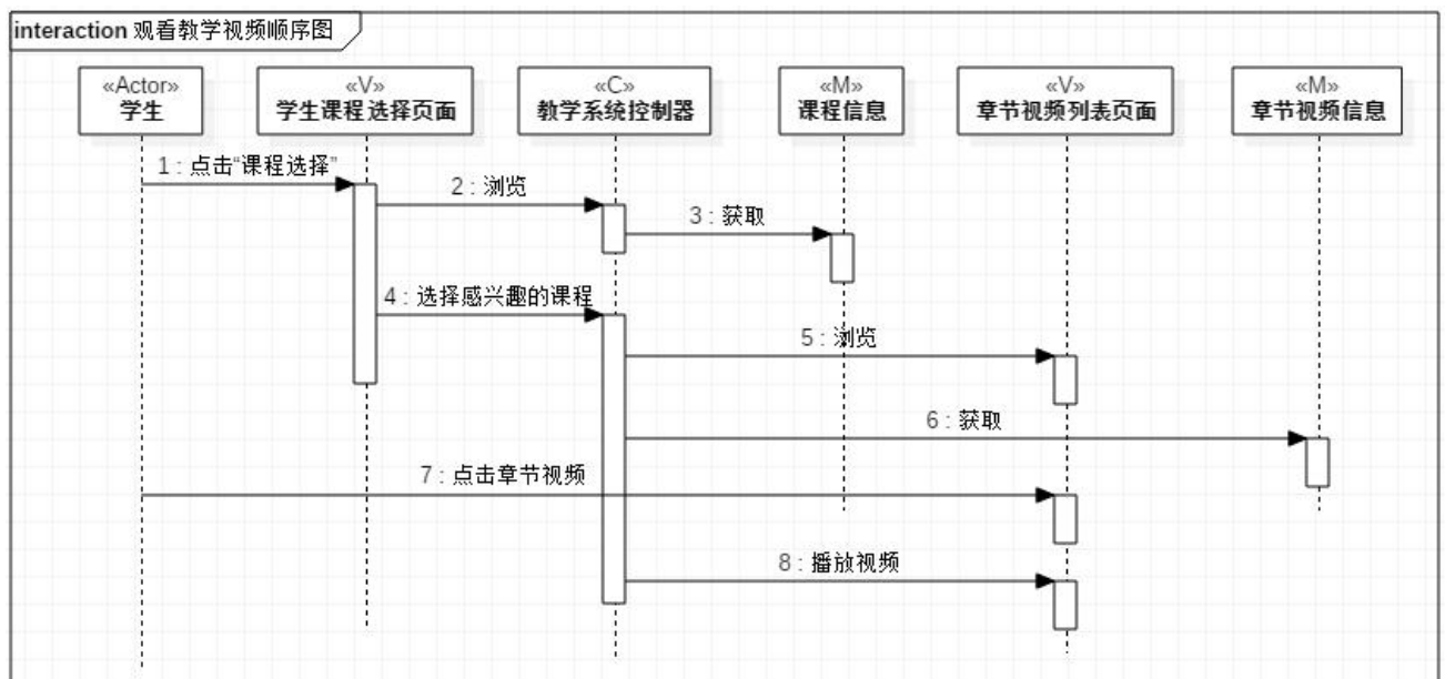
图 8 观看教学视频顺序图
