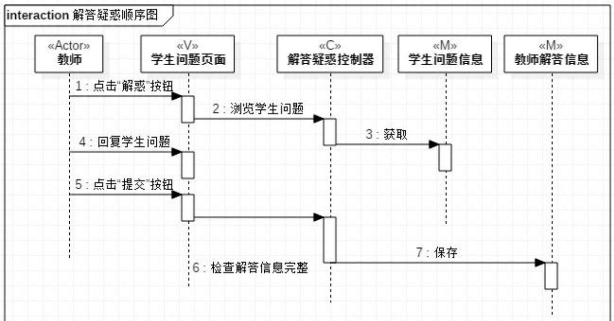
图 10 解答疑惑顺序图
