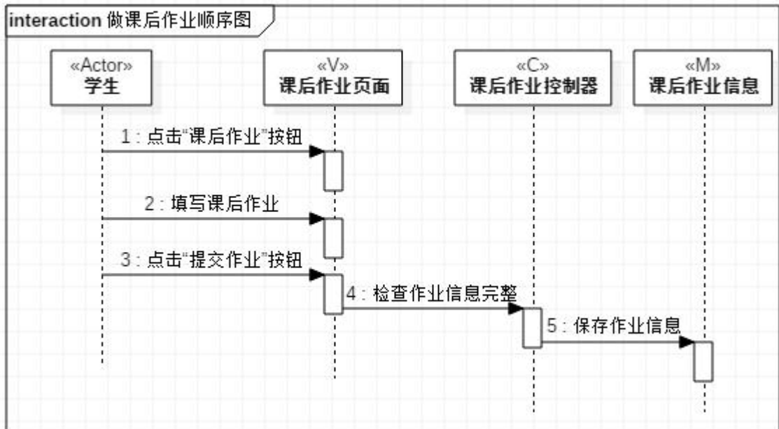
图 9 做课后作业顺序图
