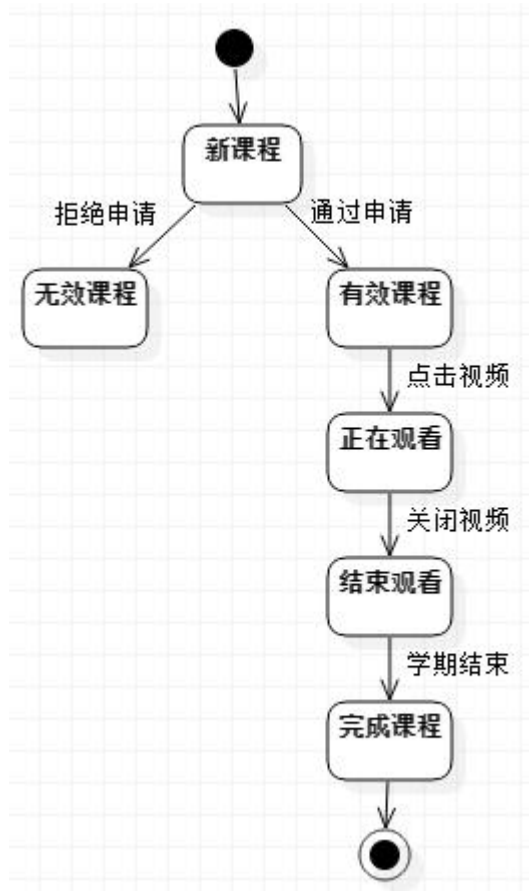
图 11 “课程” 状态图
