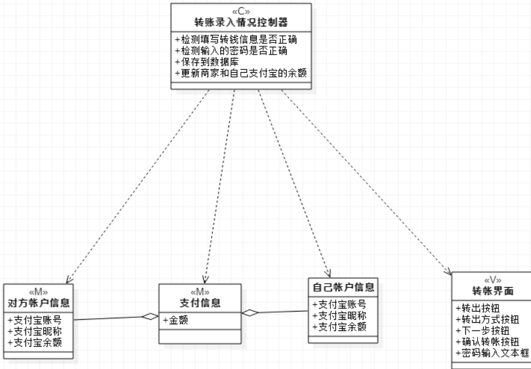
图 3：转账类图
