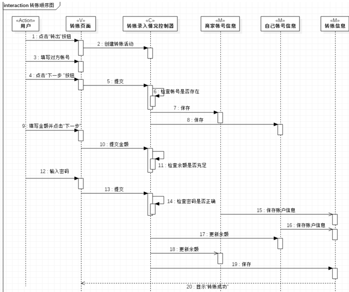
图 5：转账顺序图
