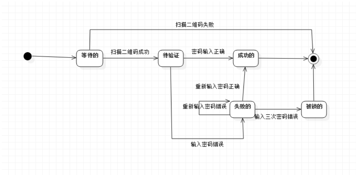
图 8：“支付” 状态图
