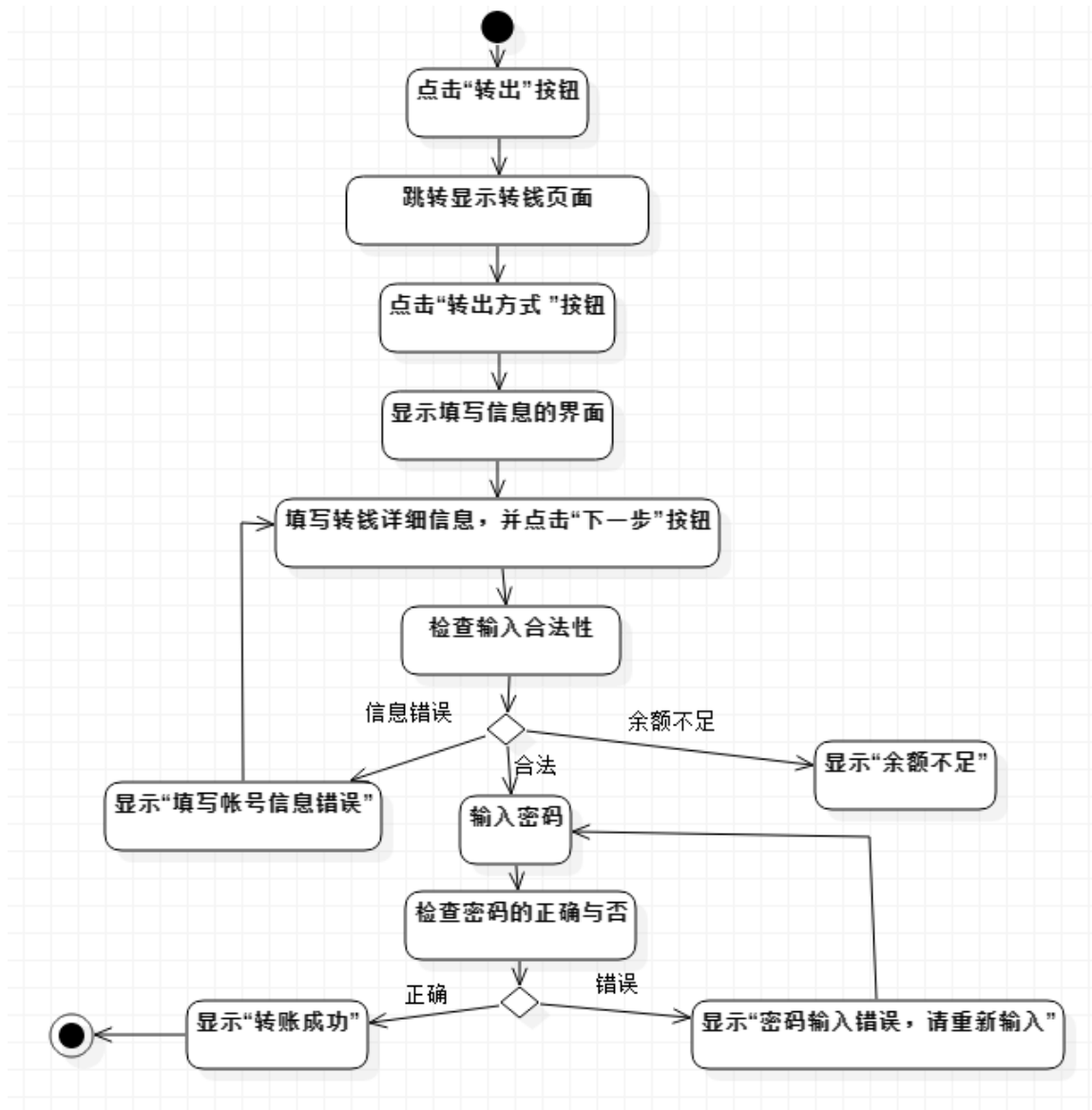
图 1:转账活动图
