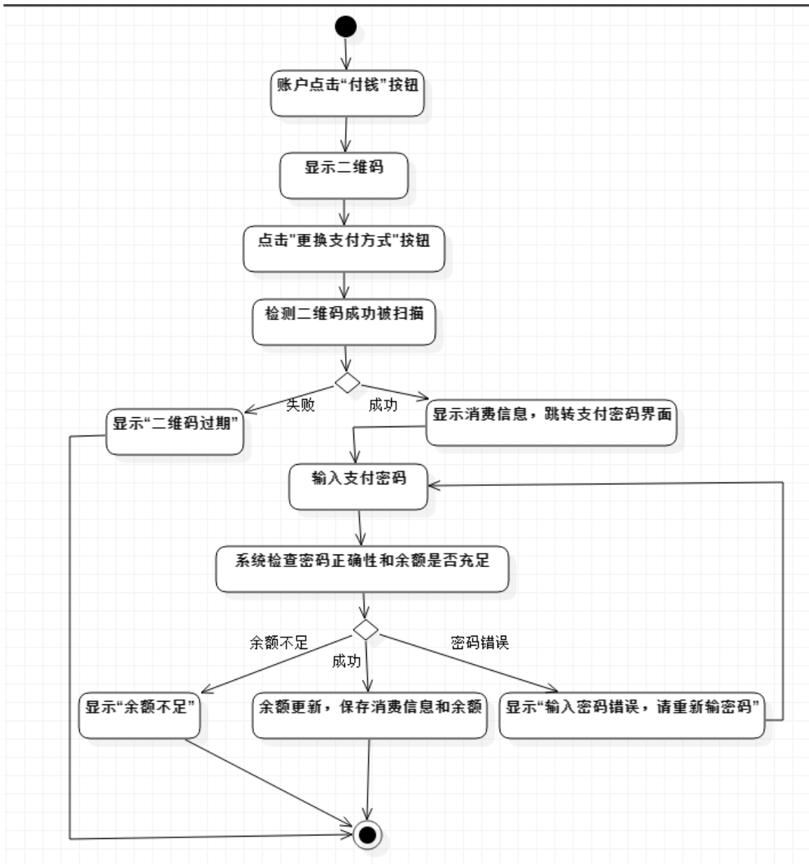
图 2:付款活动图
