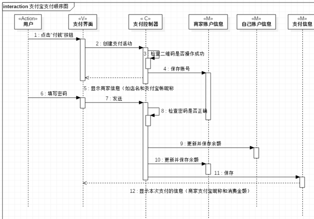
图 6：支付顺序图
