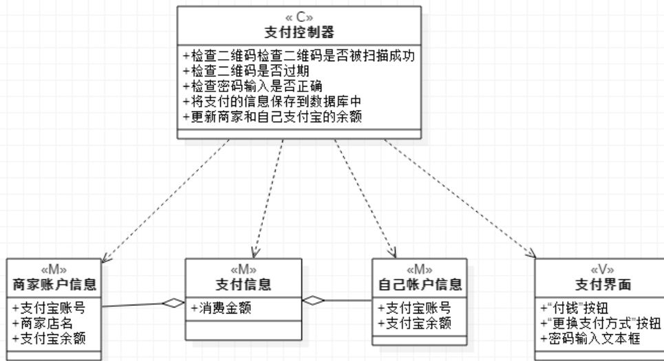
图 4：付款类图
