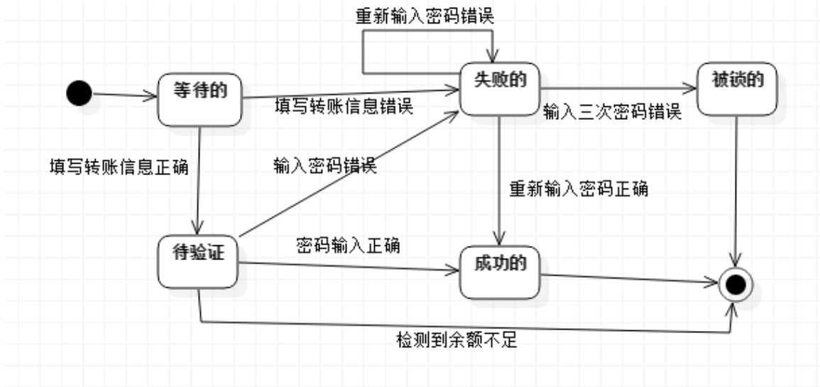
图 7：“转账” 状态图
