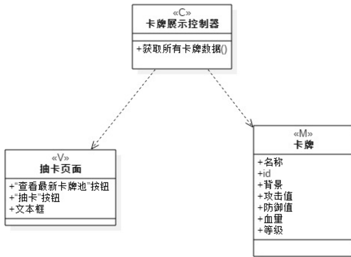
图 3.1 用例 UC001 类图
