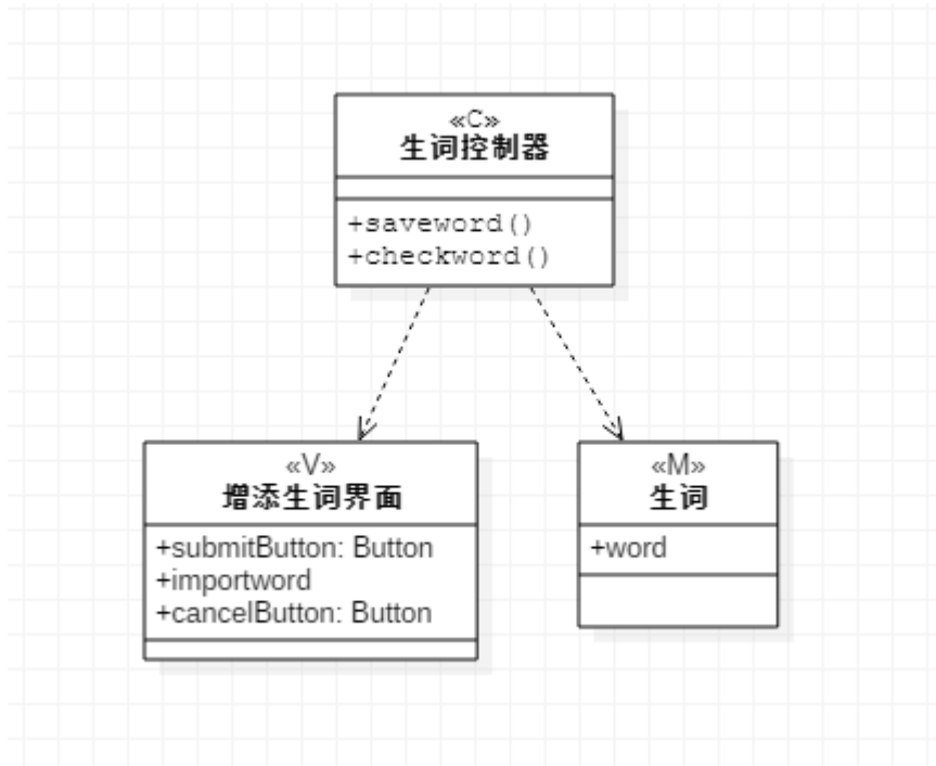
图 3: 添加生词类图
