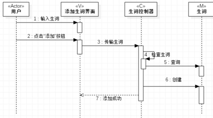
图 5: 添加生词顺序图
