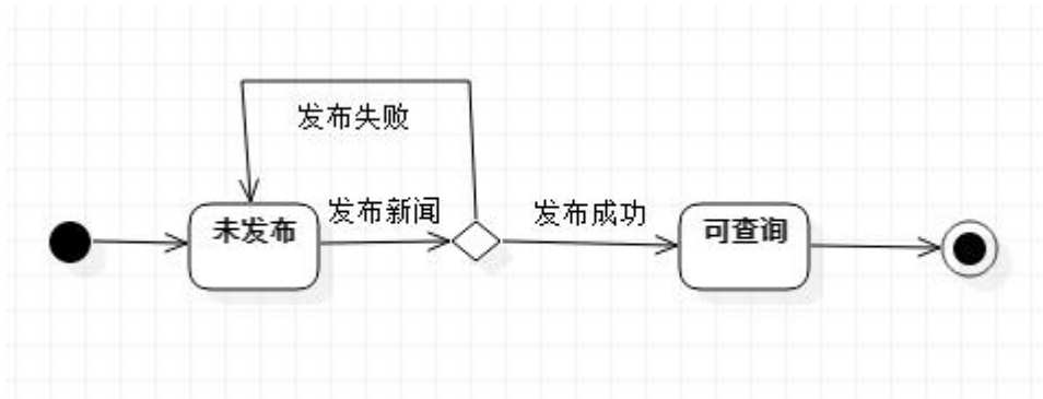
图 11: 发布新闻状态转换图
