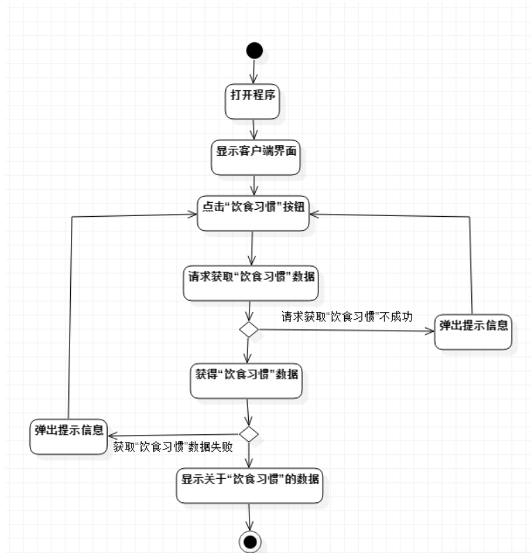
图 2-1 指导饮食习惯-活动图
