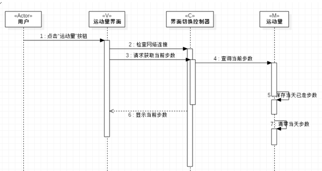
运动量交互图
