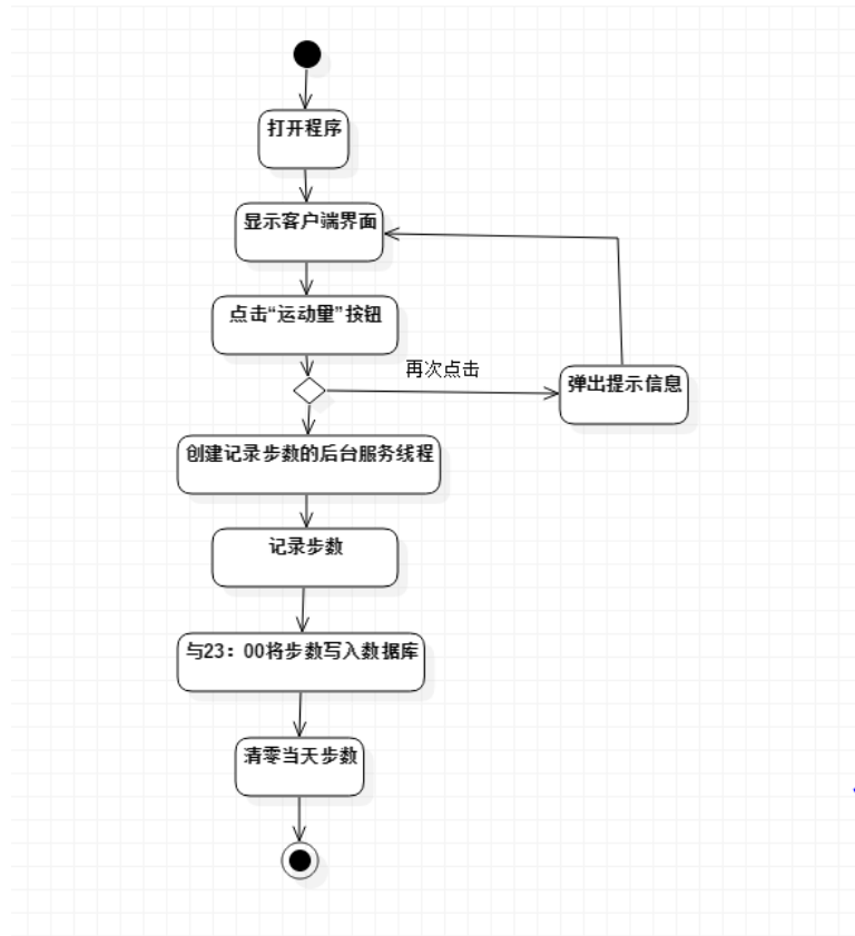
图 2-3 记录运动量-活动图
