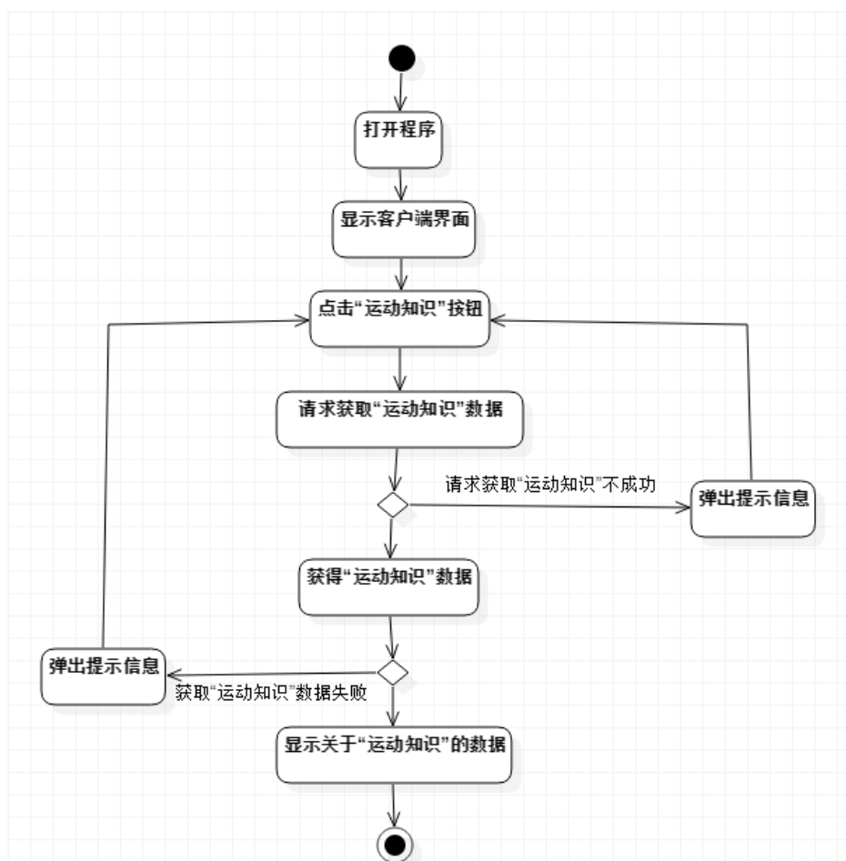
图 2-2 科普运动知识-活动图
