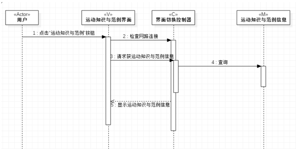
运动知识与范例模型图
