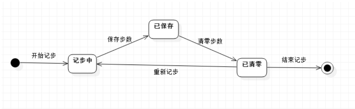
运动量状态图
