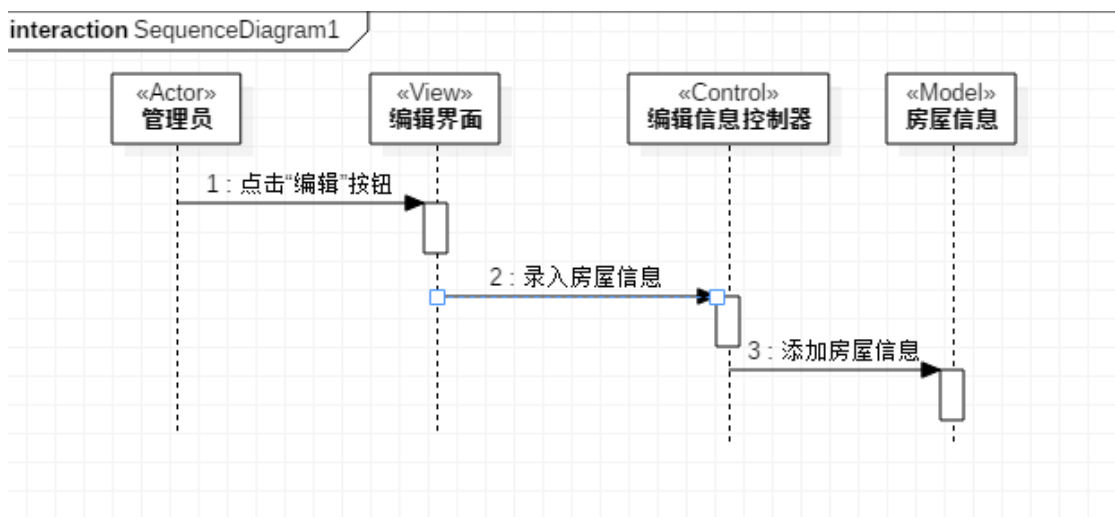
图 6: 编辑信息交互模型
