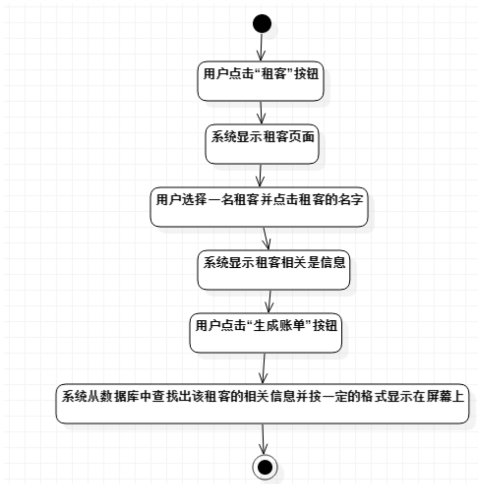
图 3：生存账单活动图
