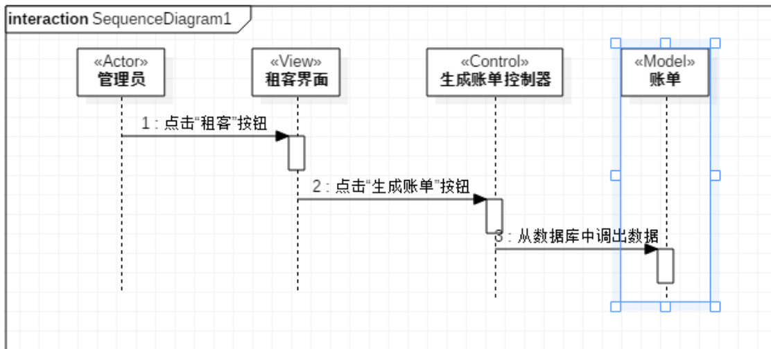
图 7：生成账单交互模型
