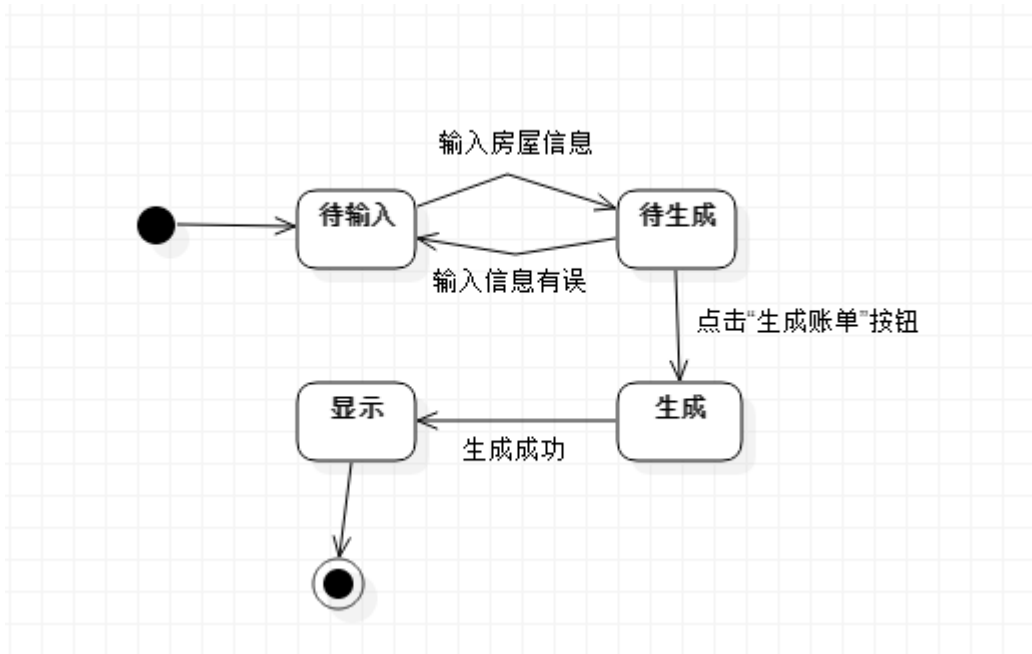
图 8：出租屋管理系统状态图
