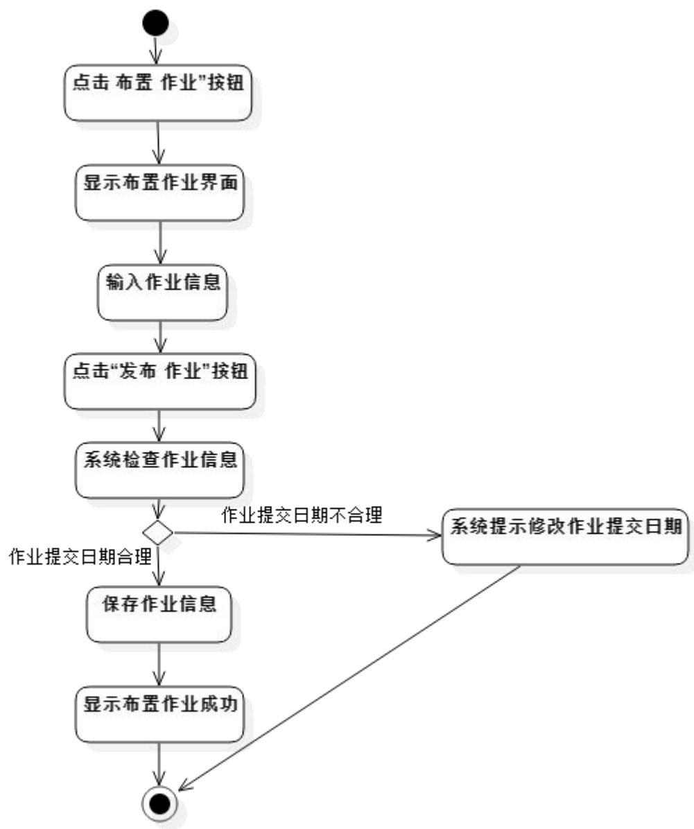
图 2：“布置作业任务”活动图
