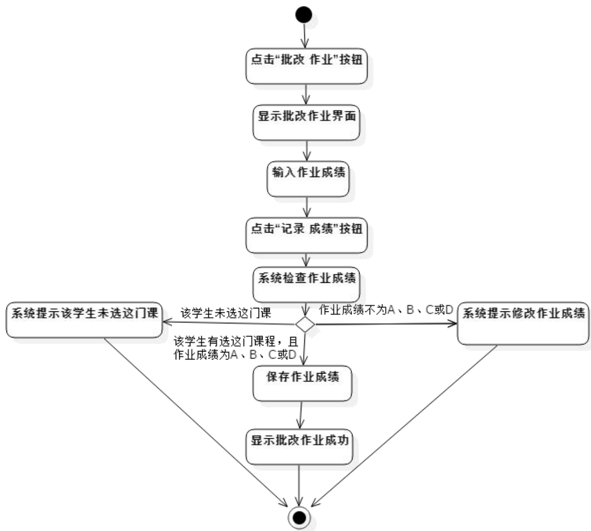
图 3：“记录作业成绩”活动图
