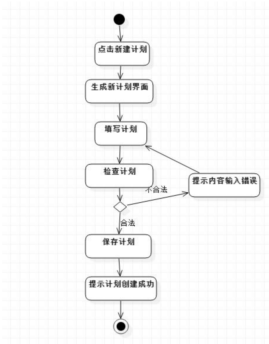
图 2: U001 活动图
