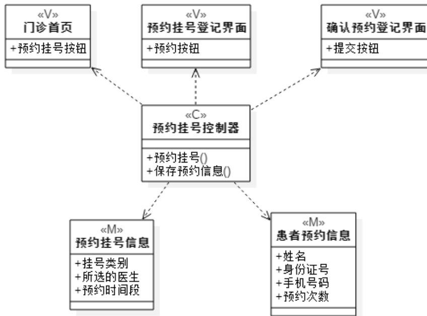
预约挂号模型
