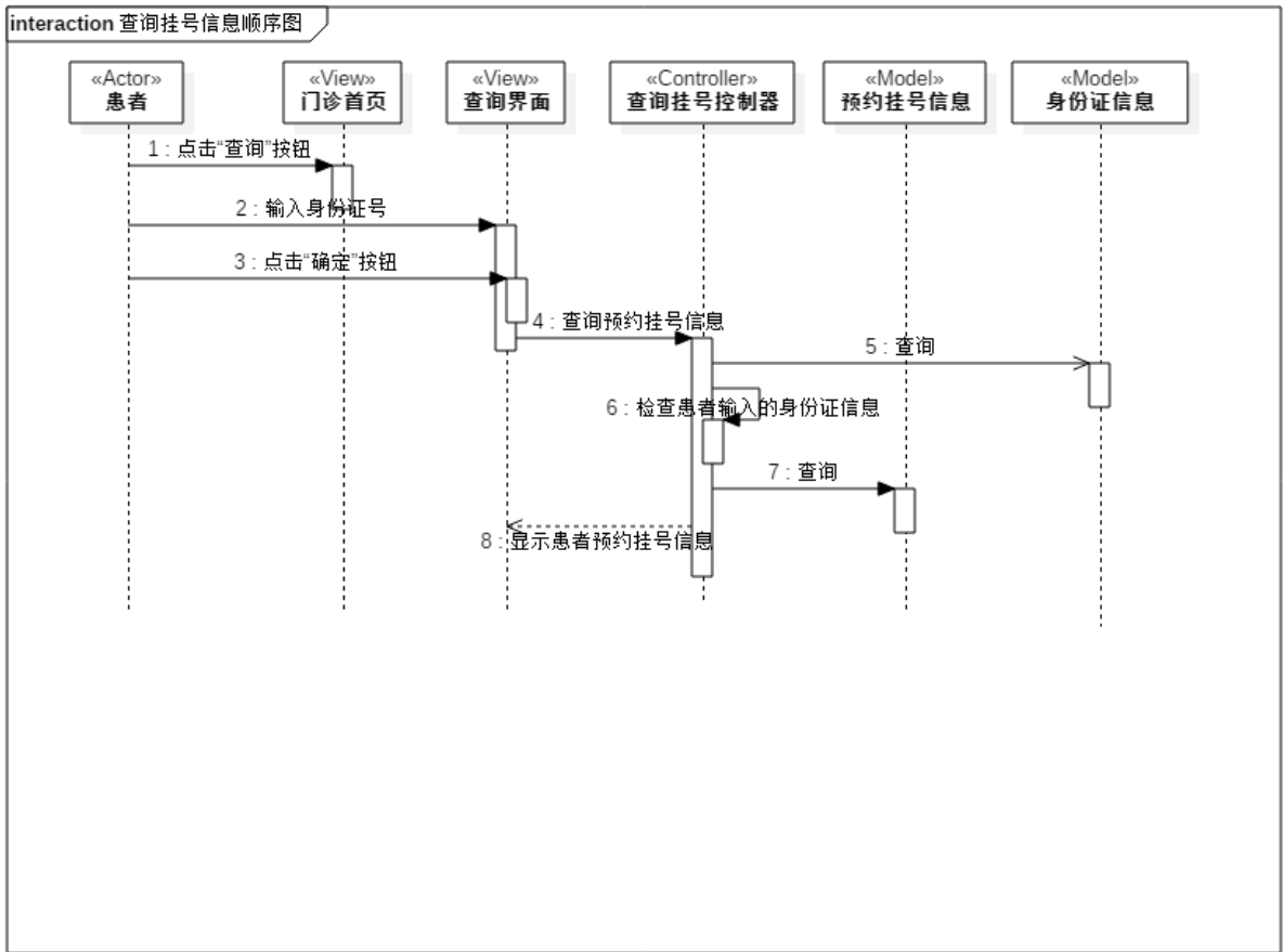
查询挂号信息顺序图
