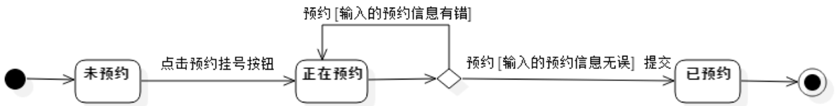
预约挂号信息状态图
