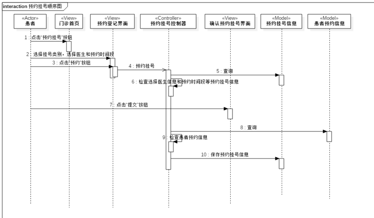
预约挂号顺序图
