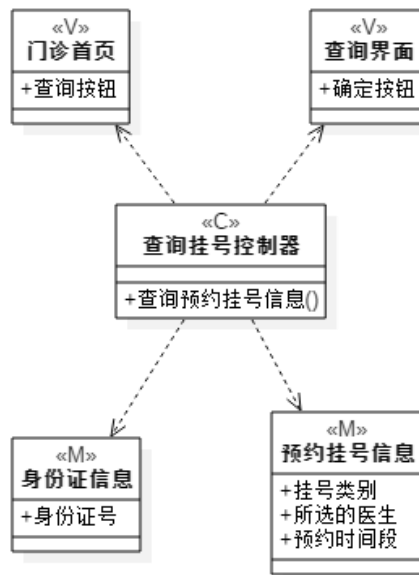
预约挂号模型
